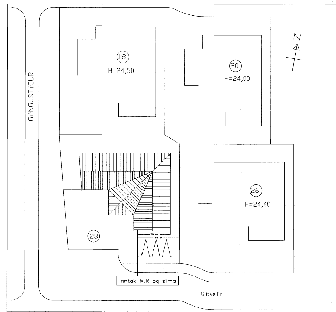
AFSTÖÐUMYND 1:500
