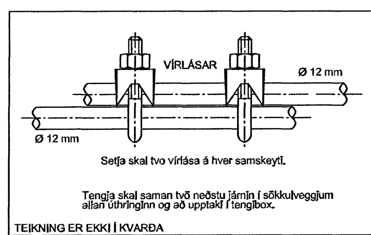
TEKNING ER EKKI Í KVARÐA SAMTENGING STEYPUPEINA DÆMIGERÐUR FRÁGANGUR
