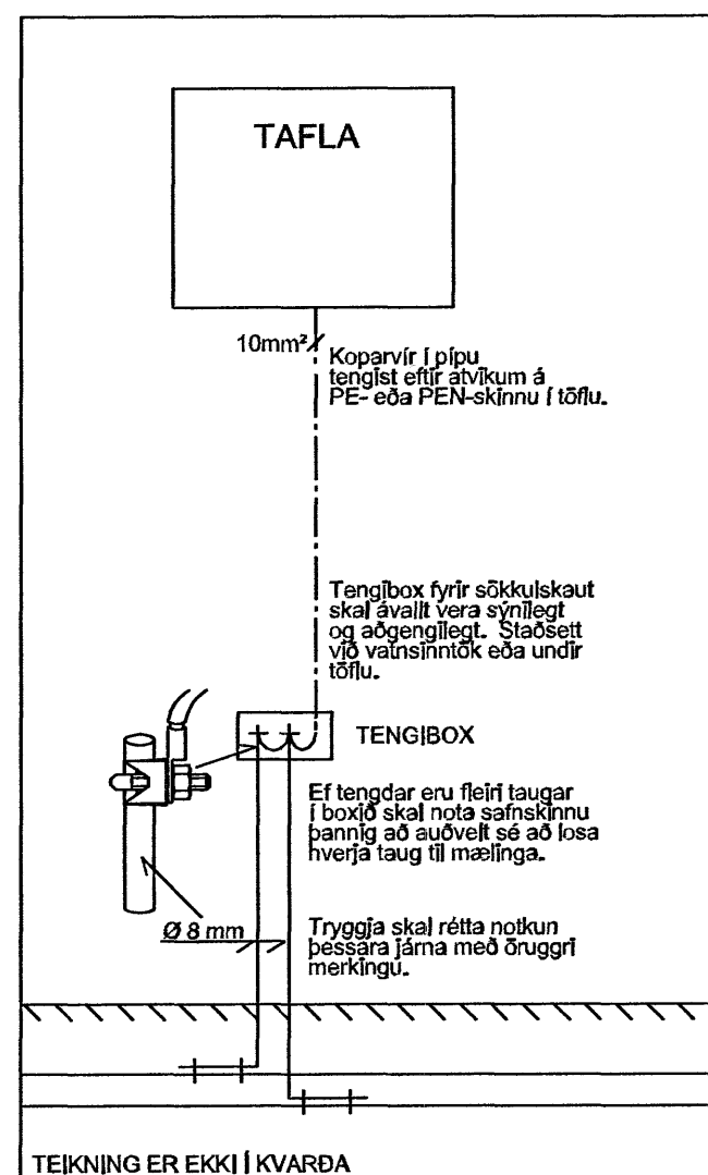
TEKNING ER EKKI Í KVARÐA SNID Í TÖFLUVEGG DÆMIGERÐUR FRÁGANGUR
