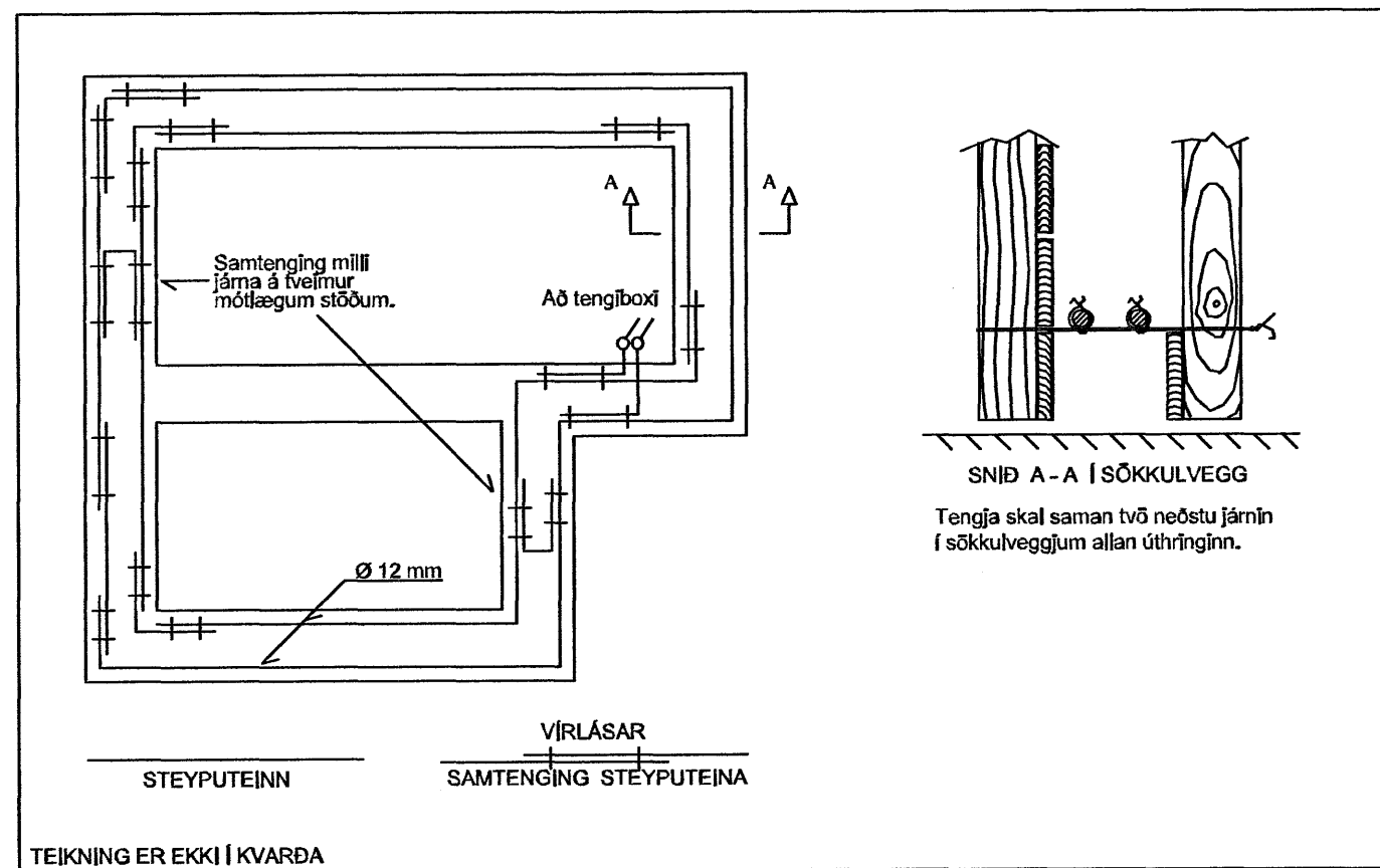
TEKNING ER EKKI Í KVARÐA FYRIRMYND GRUNNMYND SÖKKULVEGGJA DÆMIGERÐUR FRÁGANGUR
