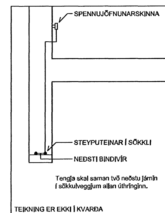
TEKNING ER EKKI Í KVARÐA ÞVERSNIÐ Í SÖKKLI DÆMIGERÐUR FRÁGANGUR
