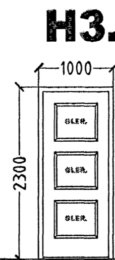
7. STK. STIGAPALLUR HURÐ OPNAST HÆGRI ÚT.
