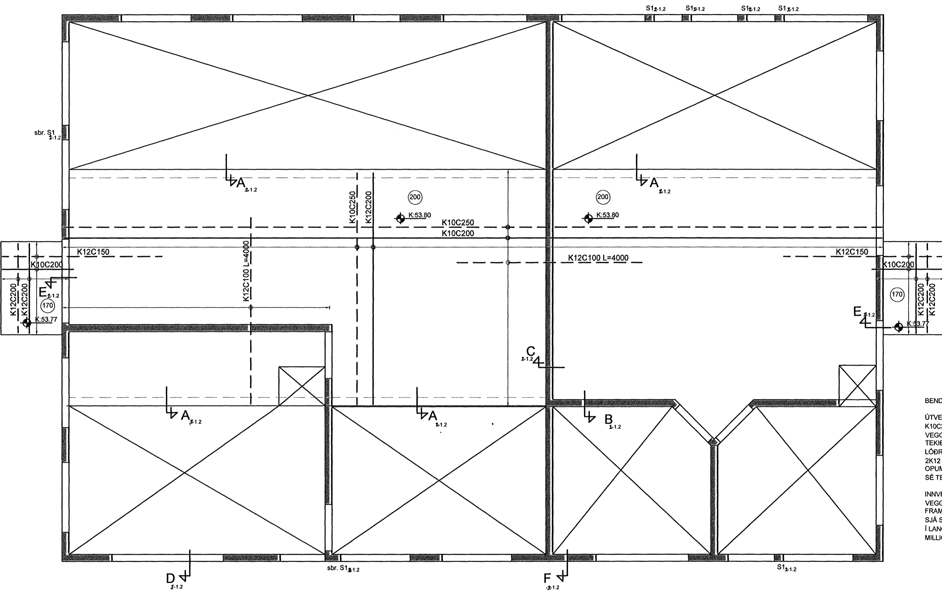
GRUNNMYND PLÖTU YFIR 1. HÆÐ, 1:50
