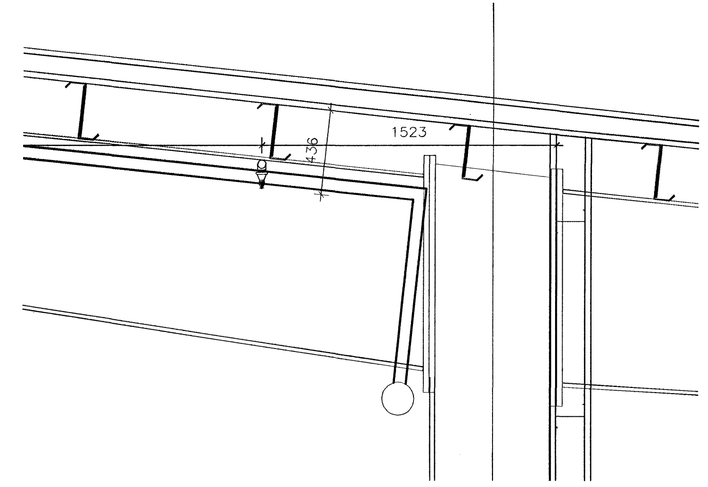
SNID A-A 1:50
