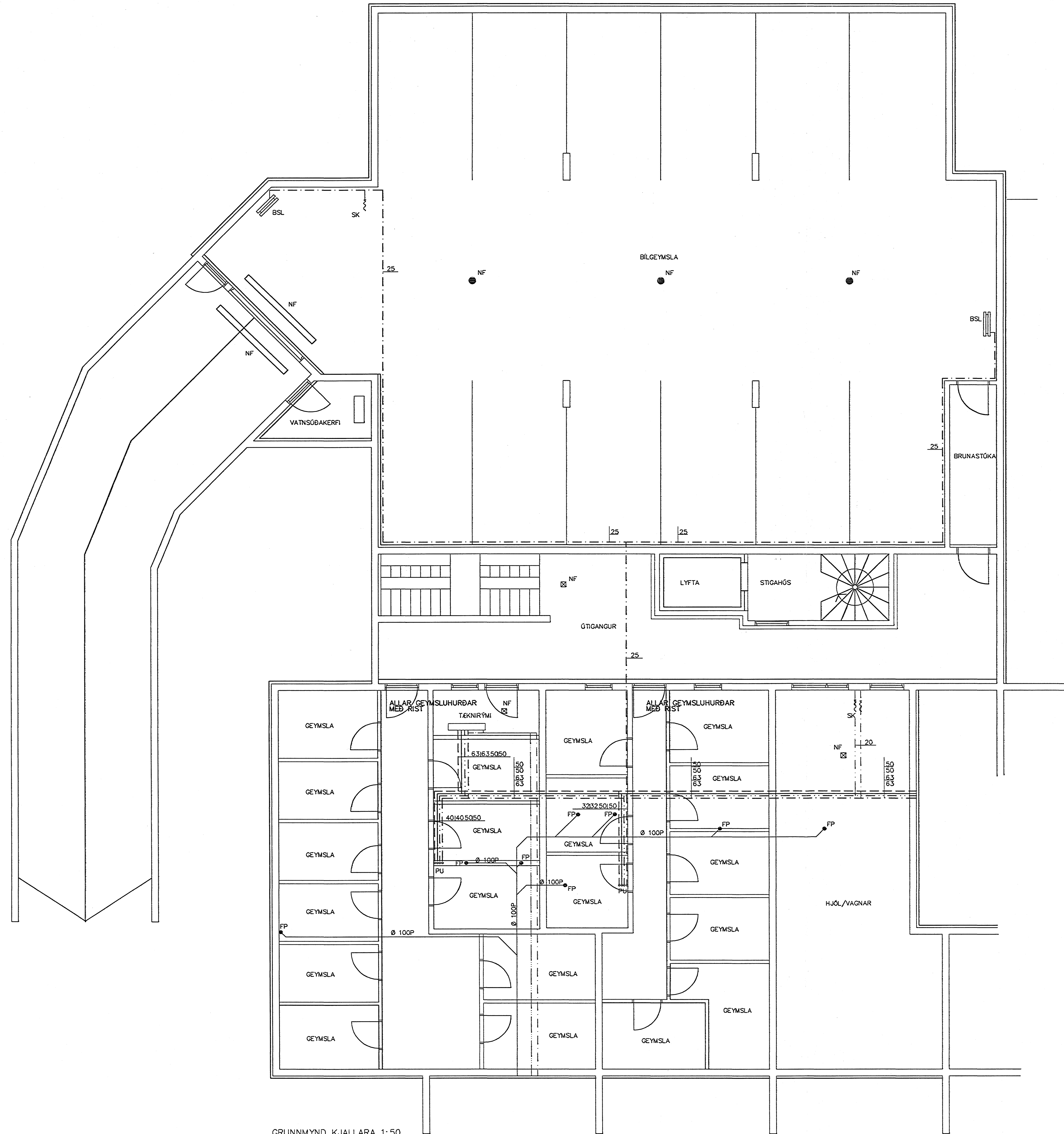
GRUNNMYND KJALLARA 1:50
