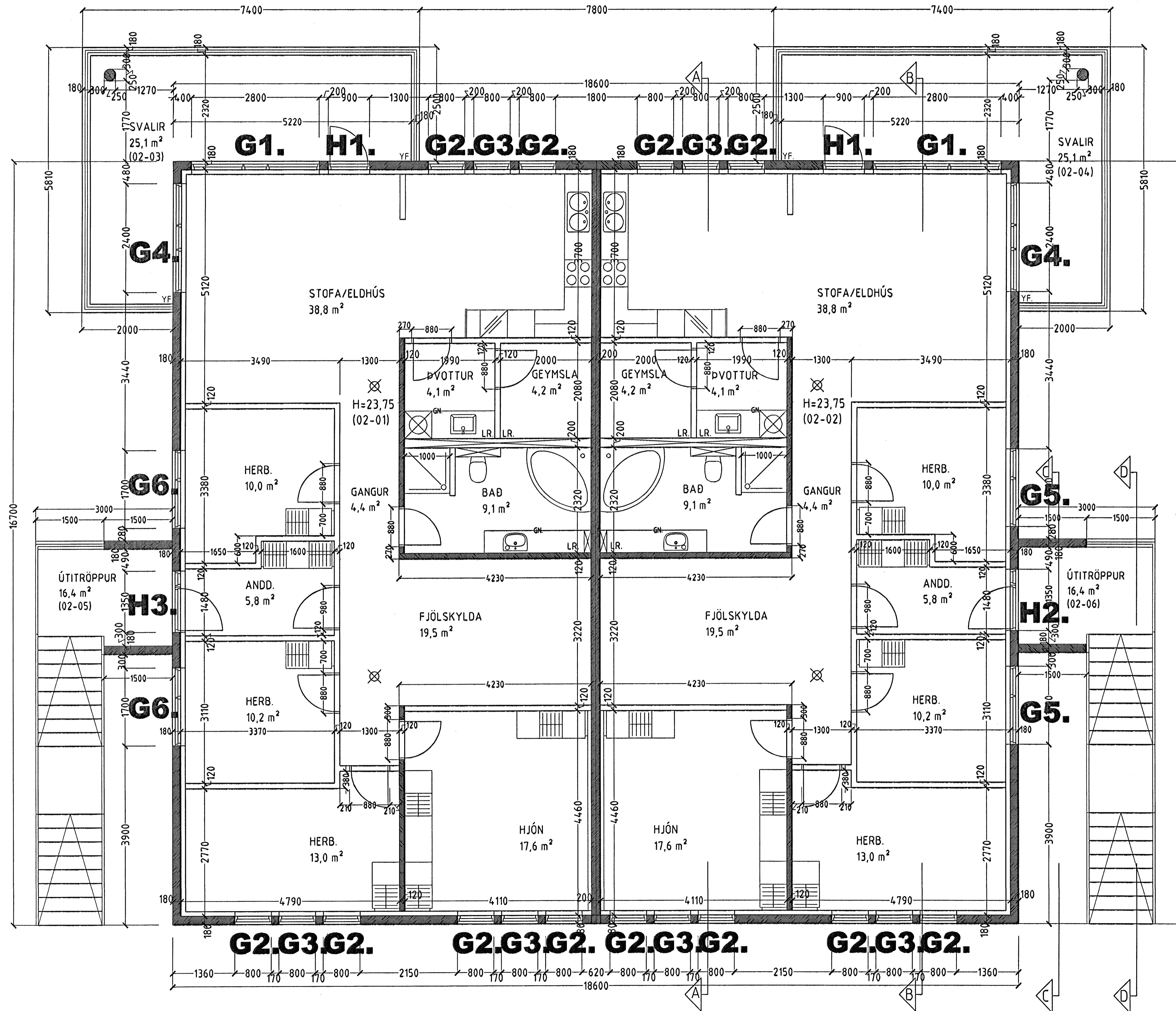
GRUNNMYND 2. HÆÐ MKV. 1:50.
