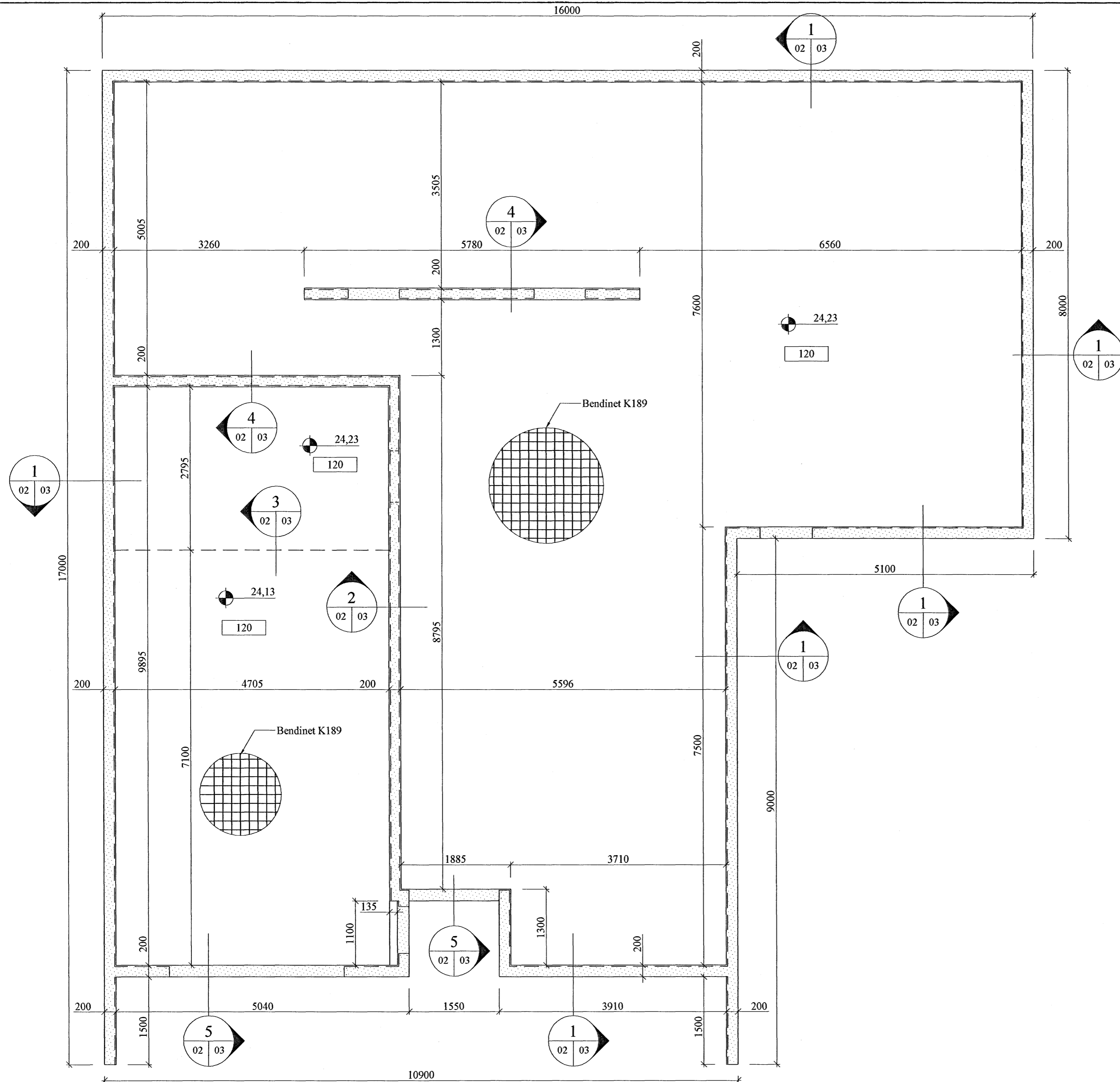
A 02 Grunnmynd undirstaða og botnplötu M 1:50
