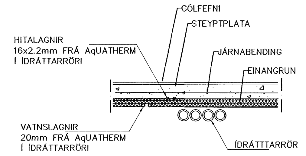
LAGNIR, SNIÐ, 1:20
