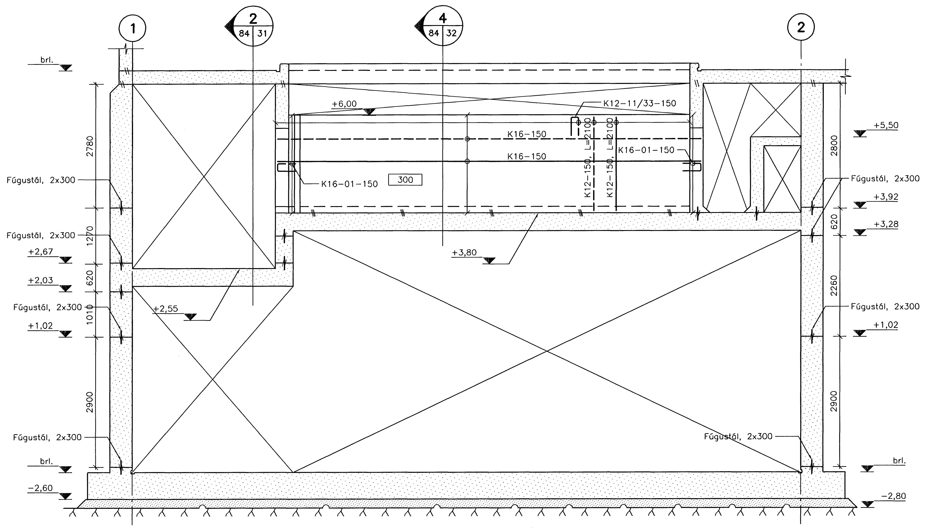
A HLIÐARMYND, VEGGUR Í MÁTLINU D +6,60 30 84 37 M. 1:50
