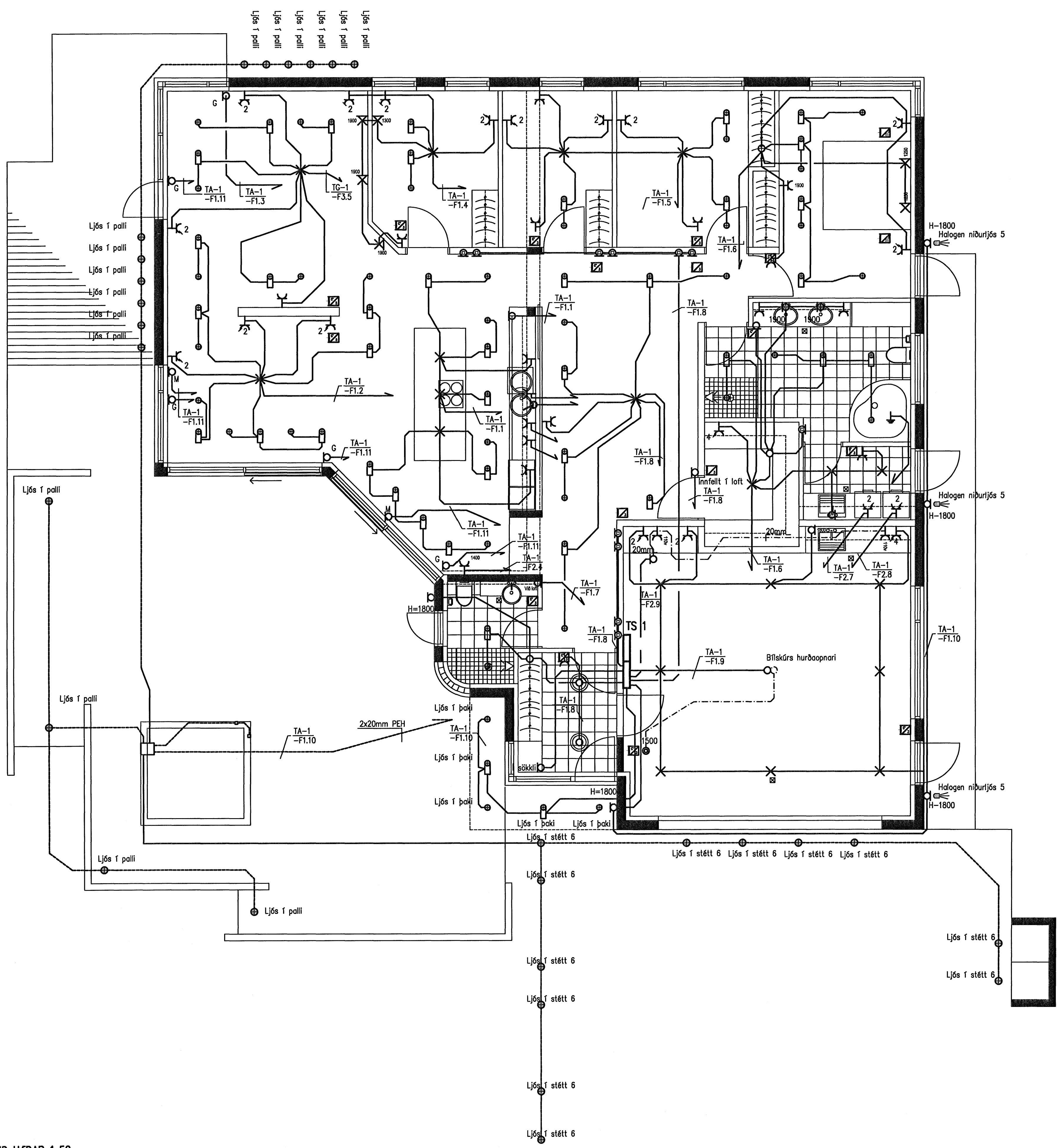
GRUNNMYND HÆÐAR 1:50
