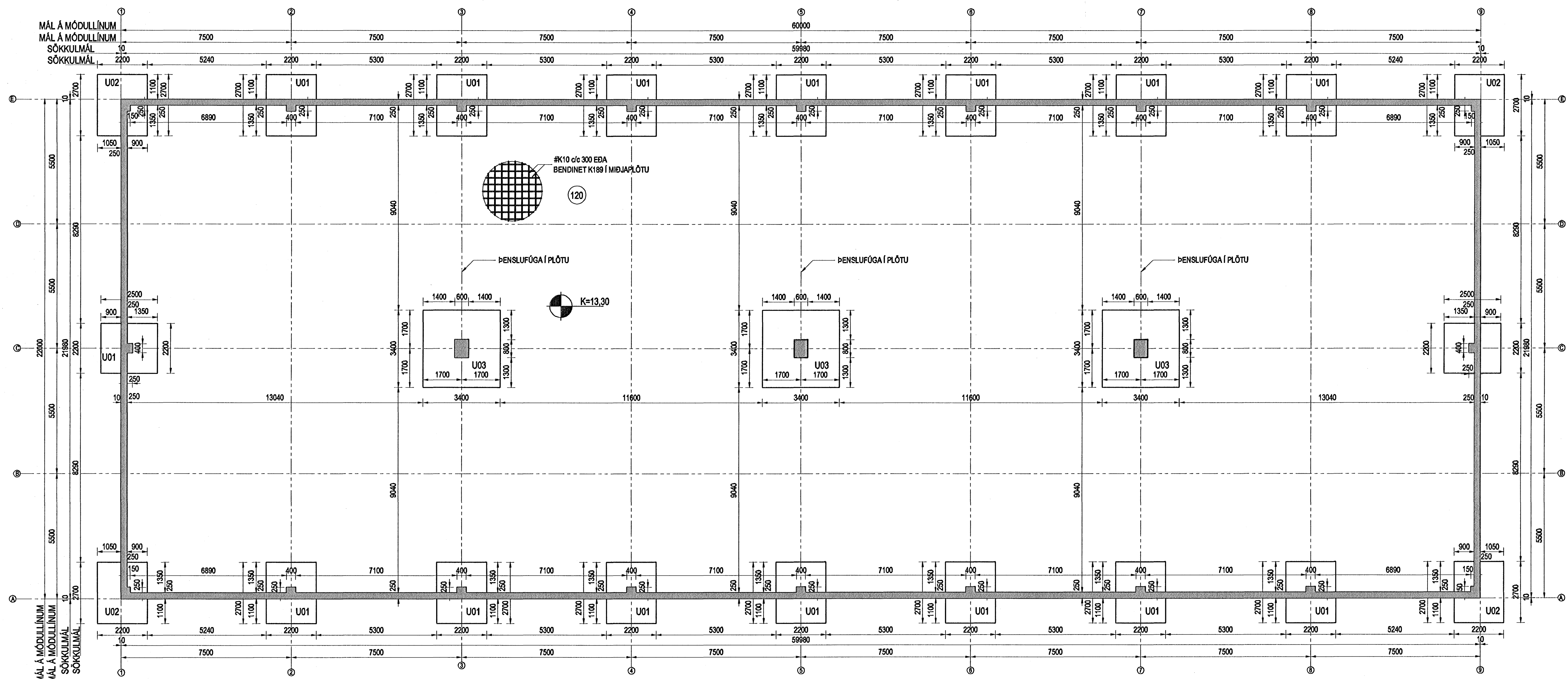
GRUNNMYND SÖKKLA MKV. 1:100
