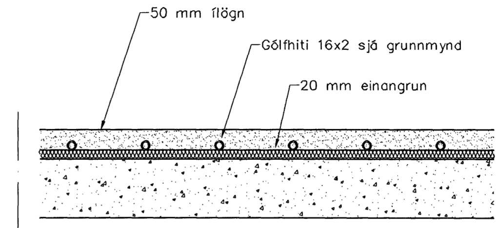
Gólfhiti. Snið 1 milliþötu, 1:10
