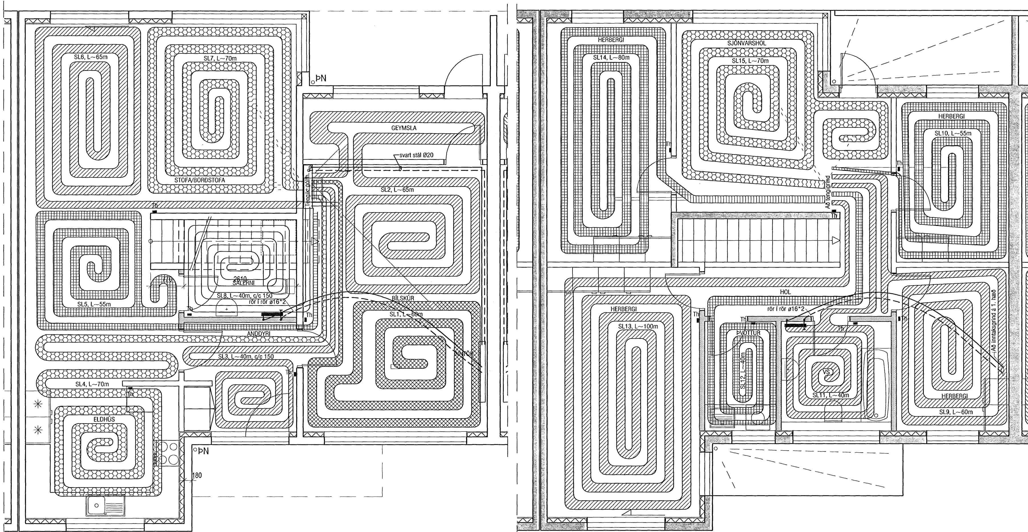
Grunnmynd 1.hæð
