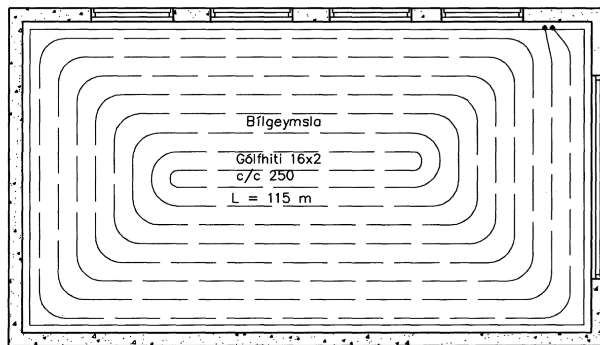
Gólfhiti, 1:50
