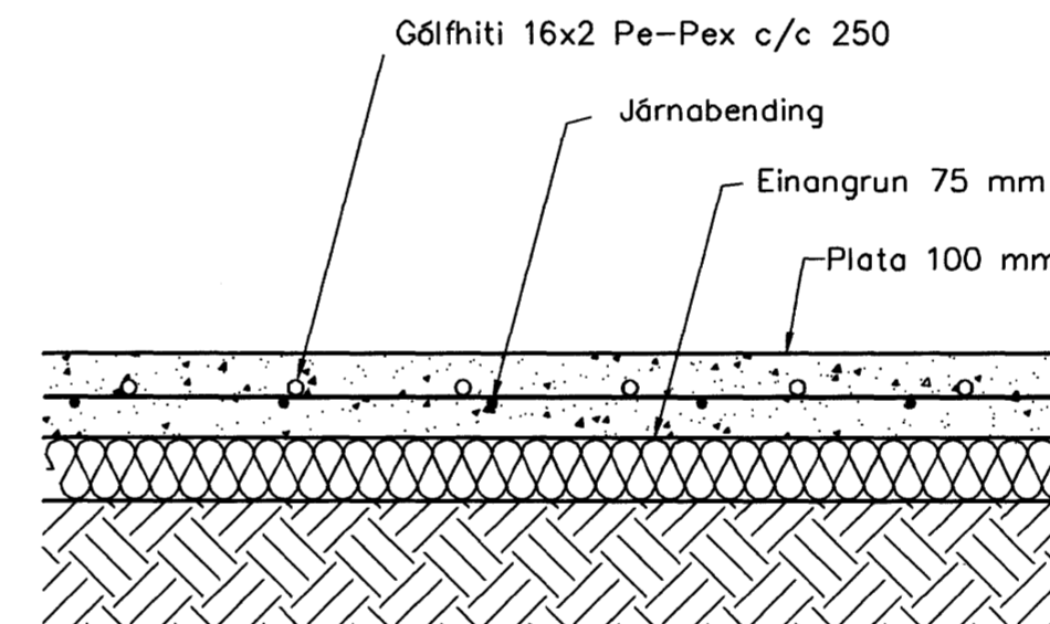
Gólfhitlagnir, Snið í botnplötu, 1:10
