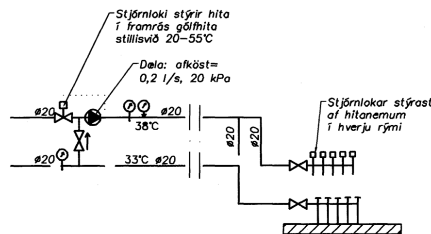
Tengigrind Gólfhita
