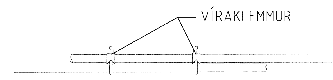
SNID AF STEYPUTEINUM Í SÖKKLUM ENGINN MÆLIKVARÐI
