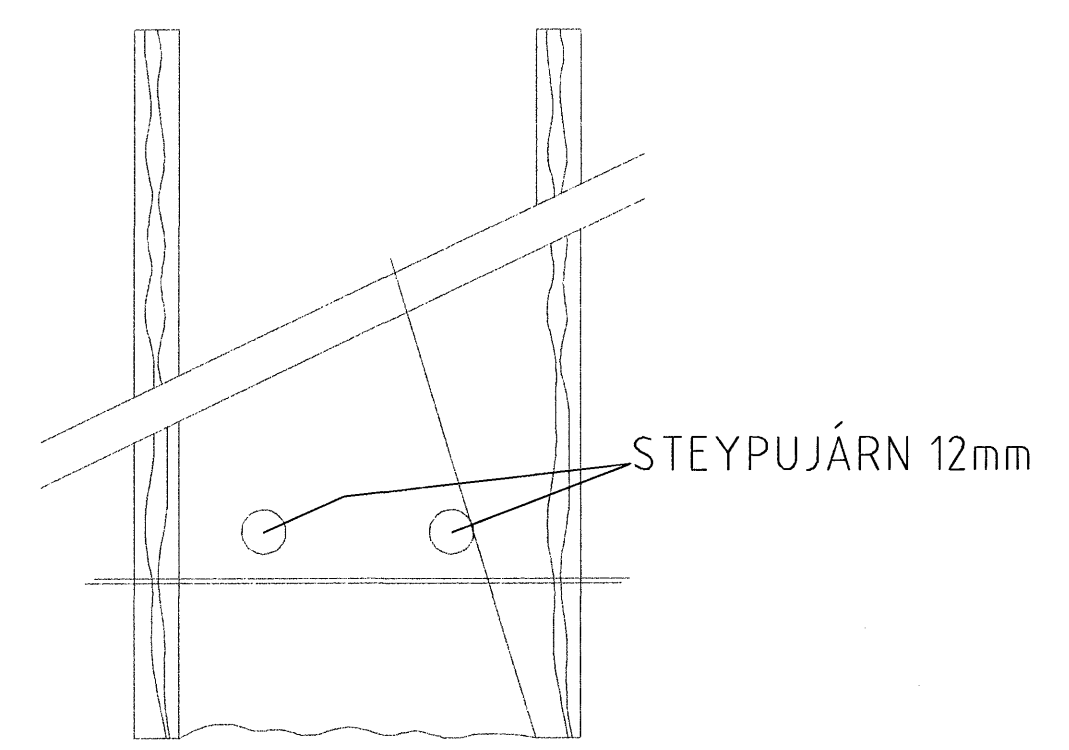
SNID AF STEYPUTEINUM Í SÖKKLUM ENGINN MÆLIKVARÐI
