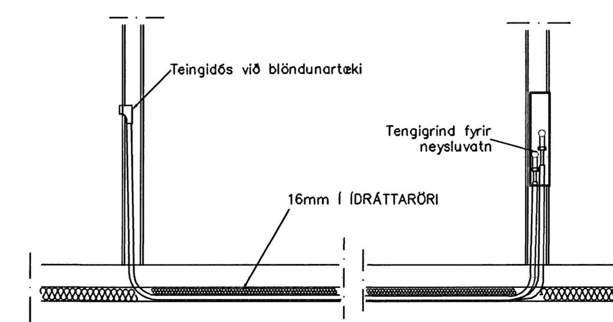
TENGING NEYSLUVATNSLAGNA 1:20
