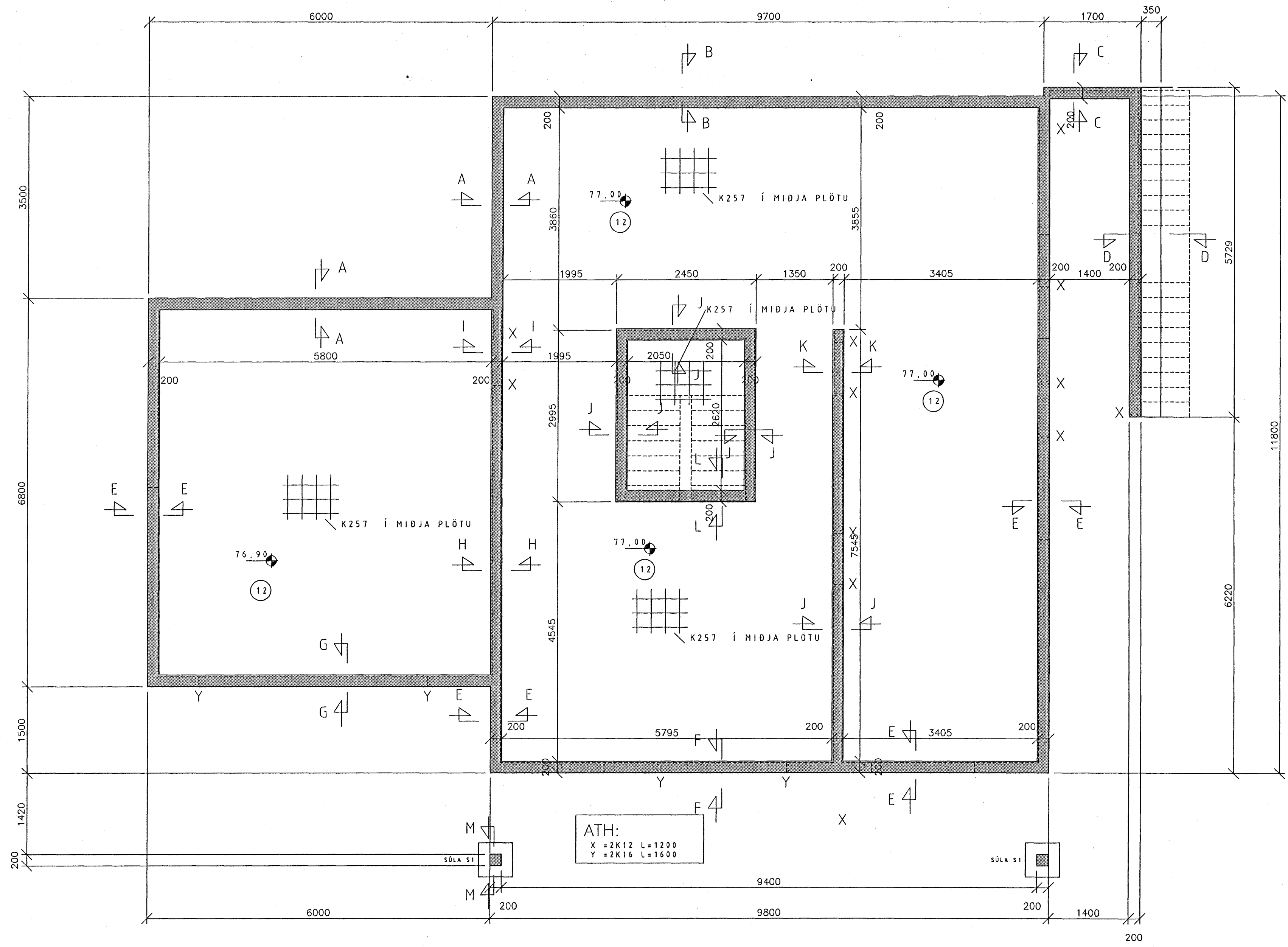
GRUNNMYND SÖKKLAR 1:50
