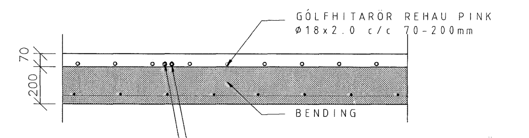
SNID, GÖLFHITALAGNIR Í ÍBÚÐ 1:20
