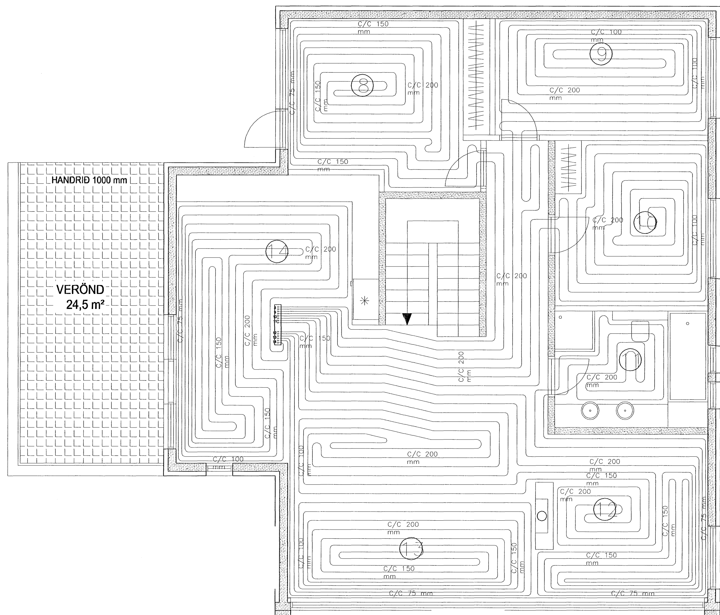
GRUNNMYND GÖLFHITALAGNA 2. HÆÐAR 1:50
