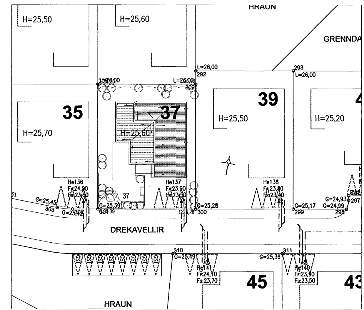
AFSTÖÐUMYND 1:500
