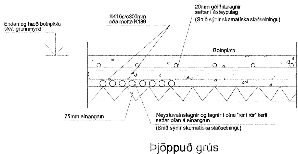
Almennt snið í botnplötu
