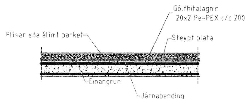
GÓLFHITI EFRIHÆÐ, SNIÐ 1:20
