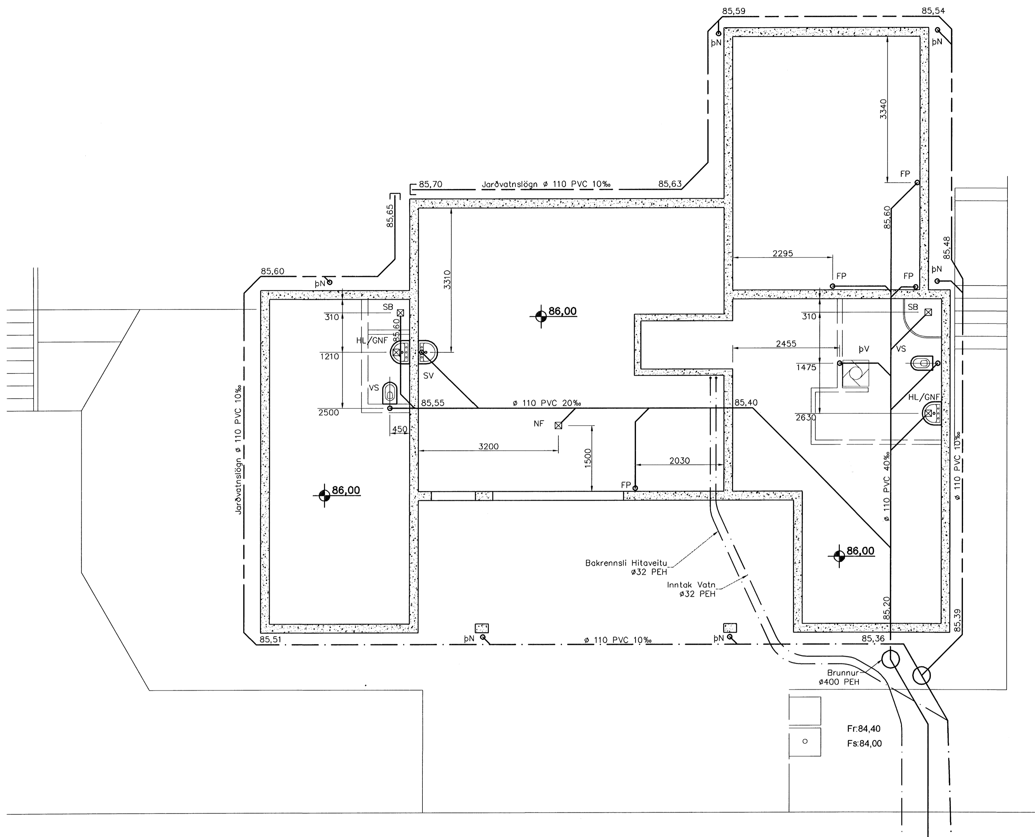
Grunnlagir 1:50
