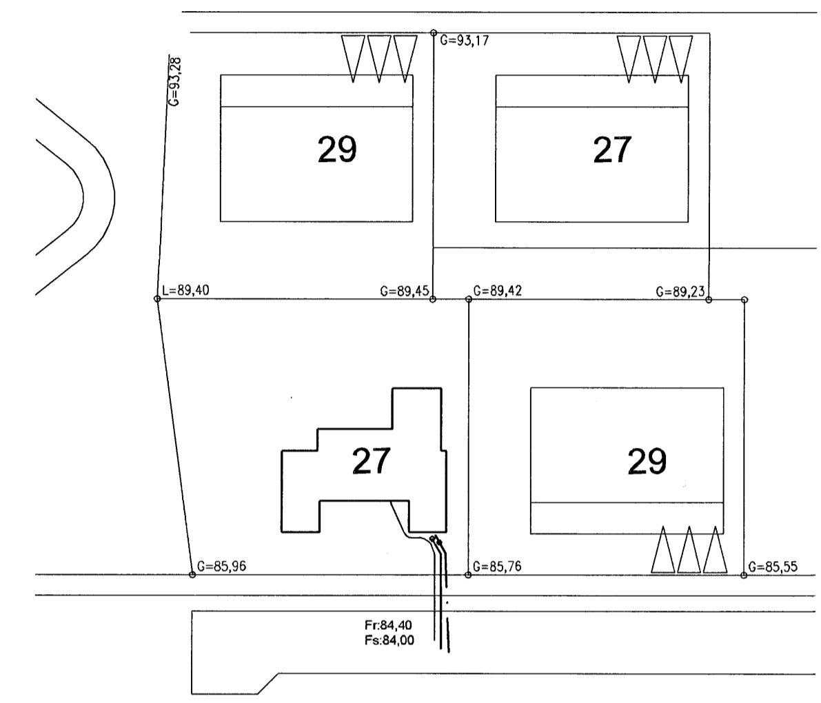
Afstöðumynd 1:50
