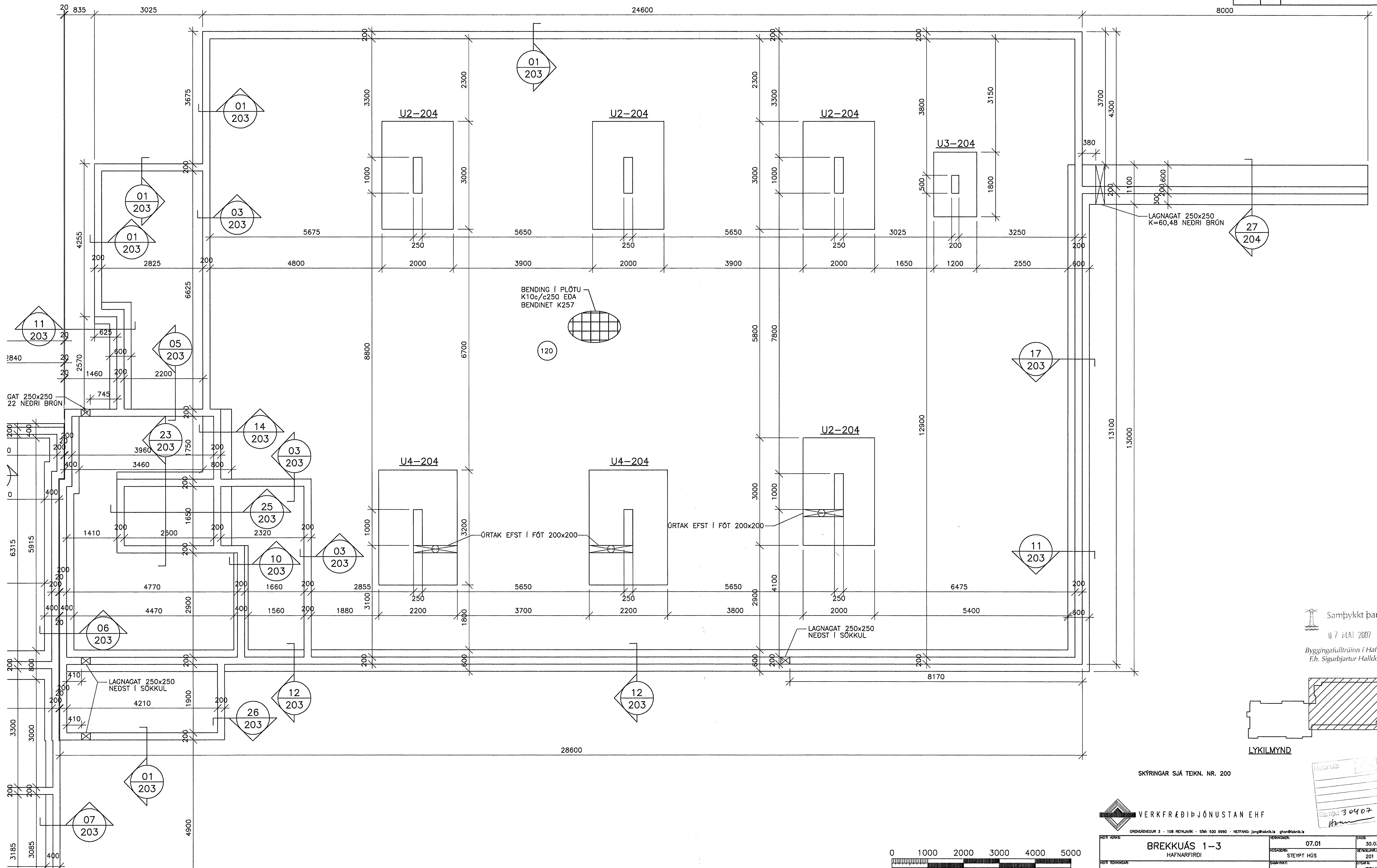
GRUNNMYND SÖKKLA. 1:50
