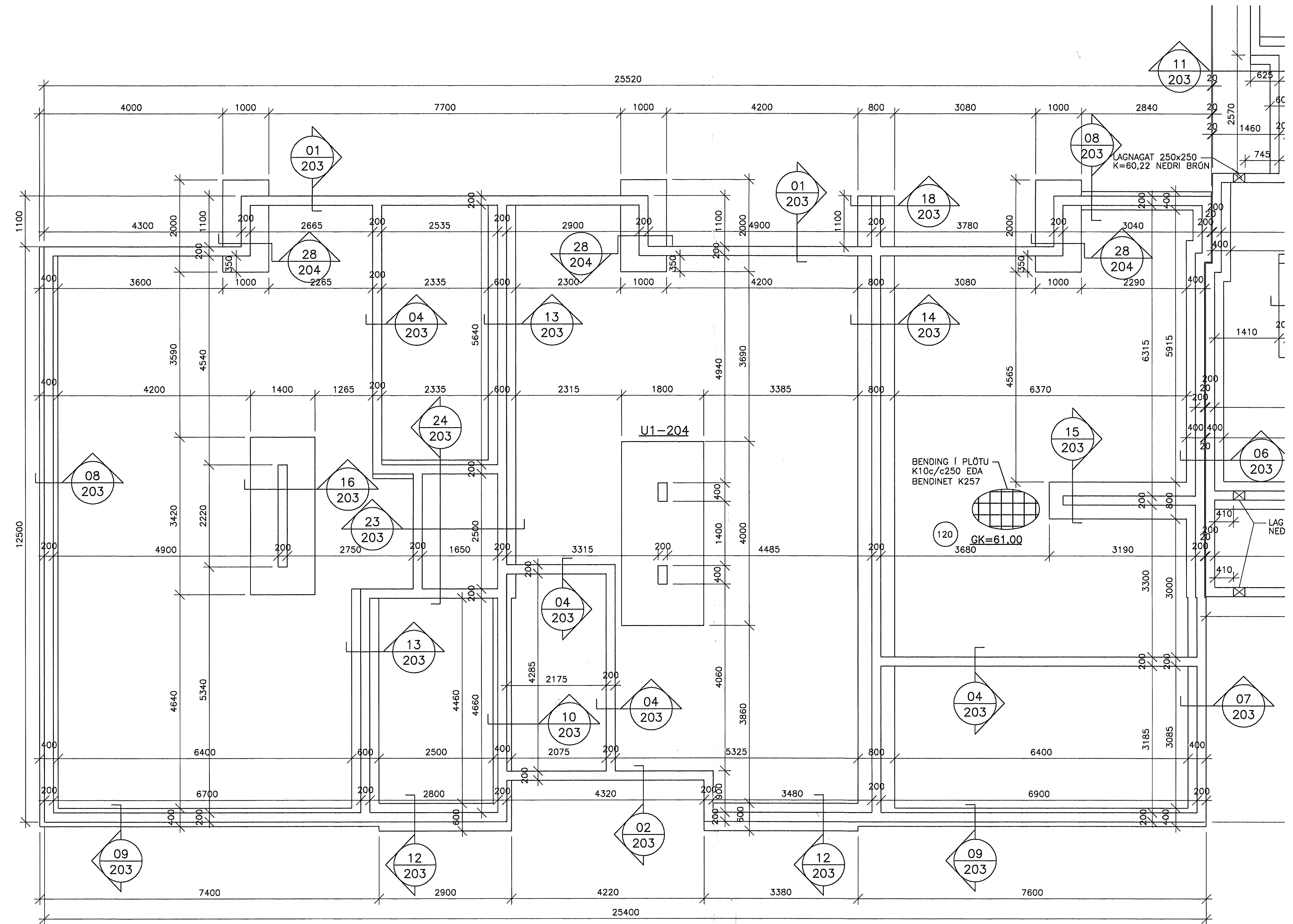
GRUNNMYND SÖKKLA, 1:50
