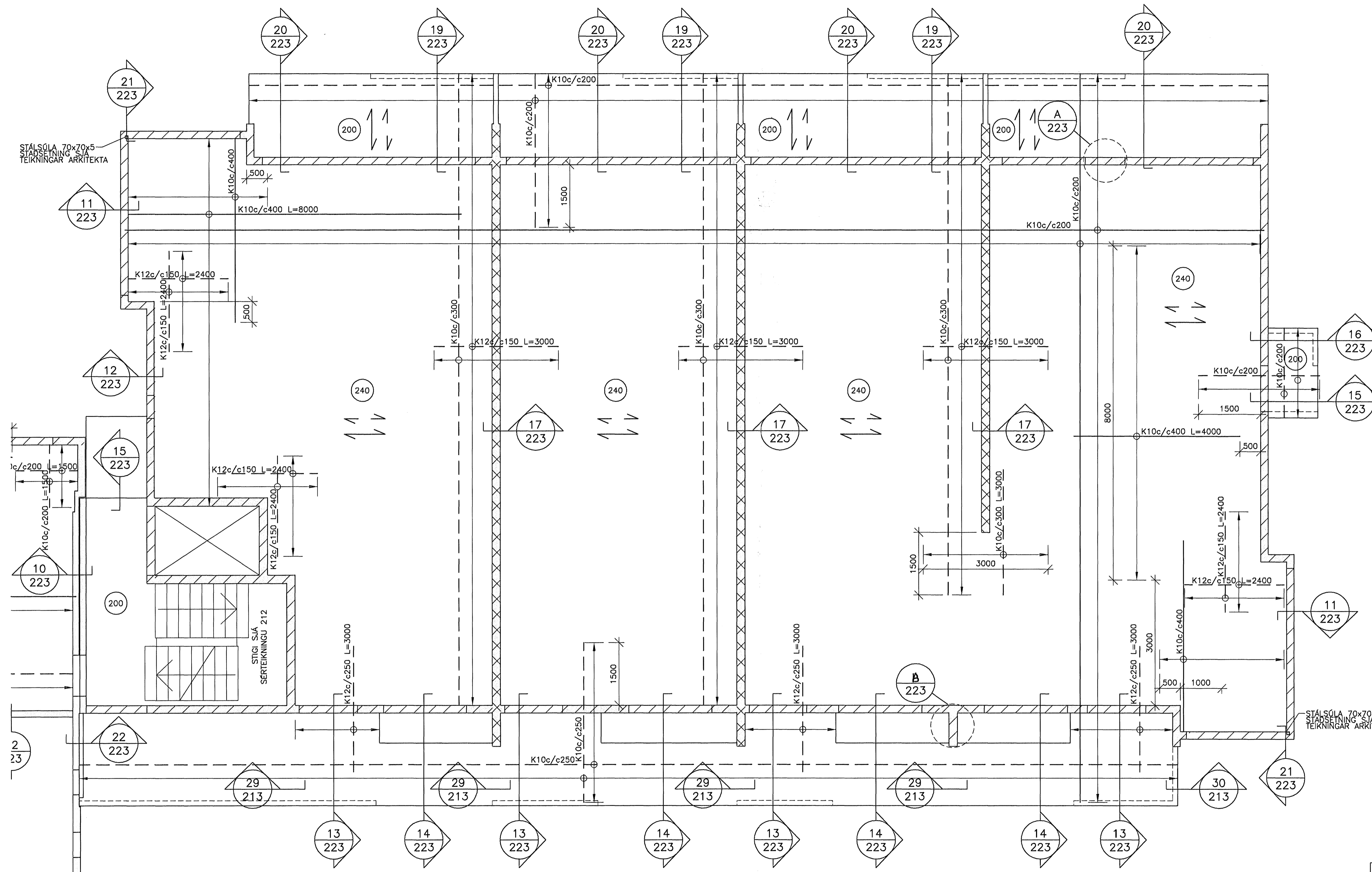
GRUNNMYND 2-3.HÆÐAR. 1:50
