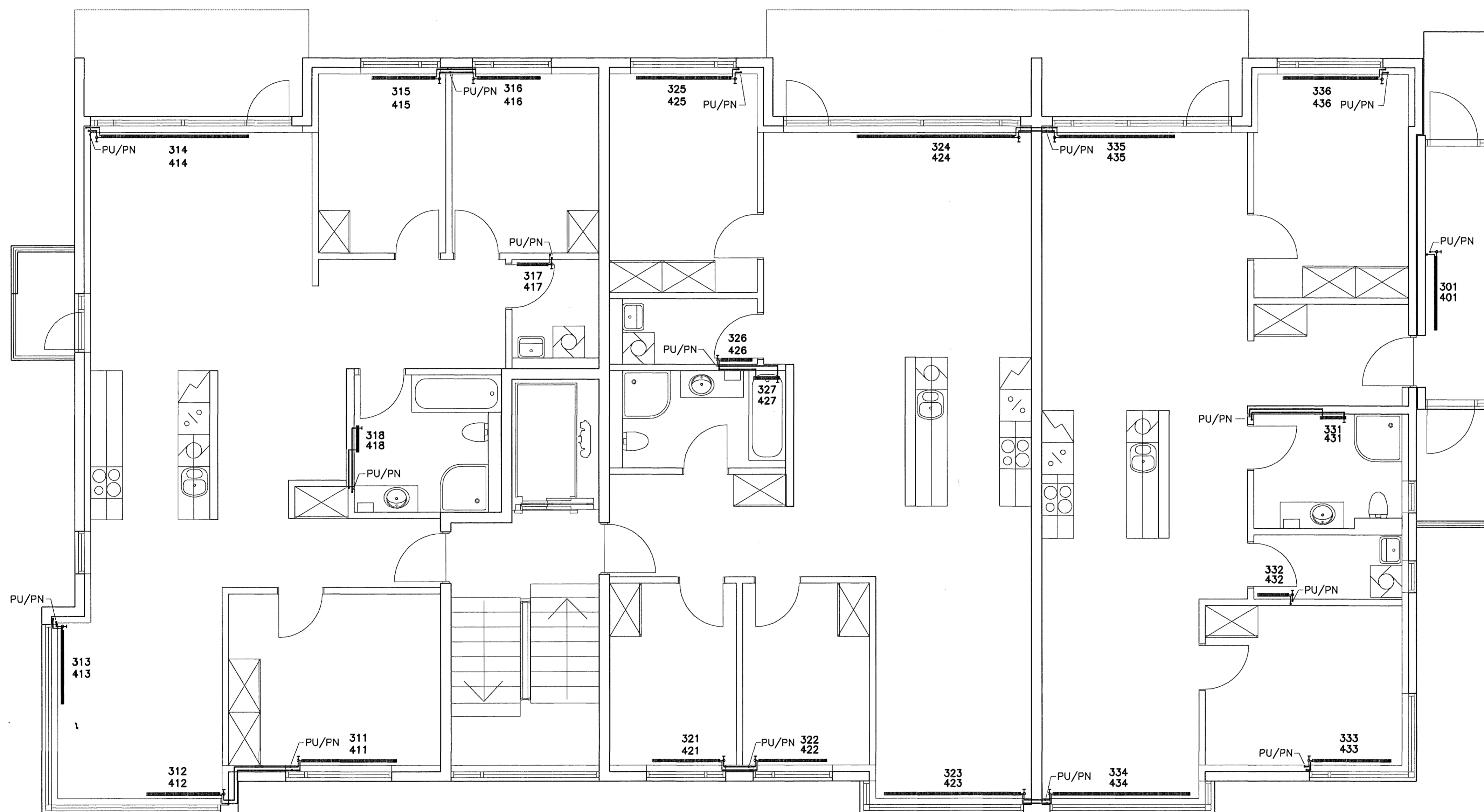
GRUNNMYND 3.-4.HÆÐ. 1:50
