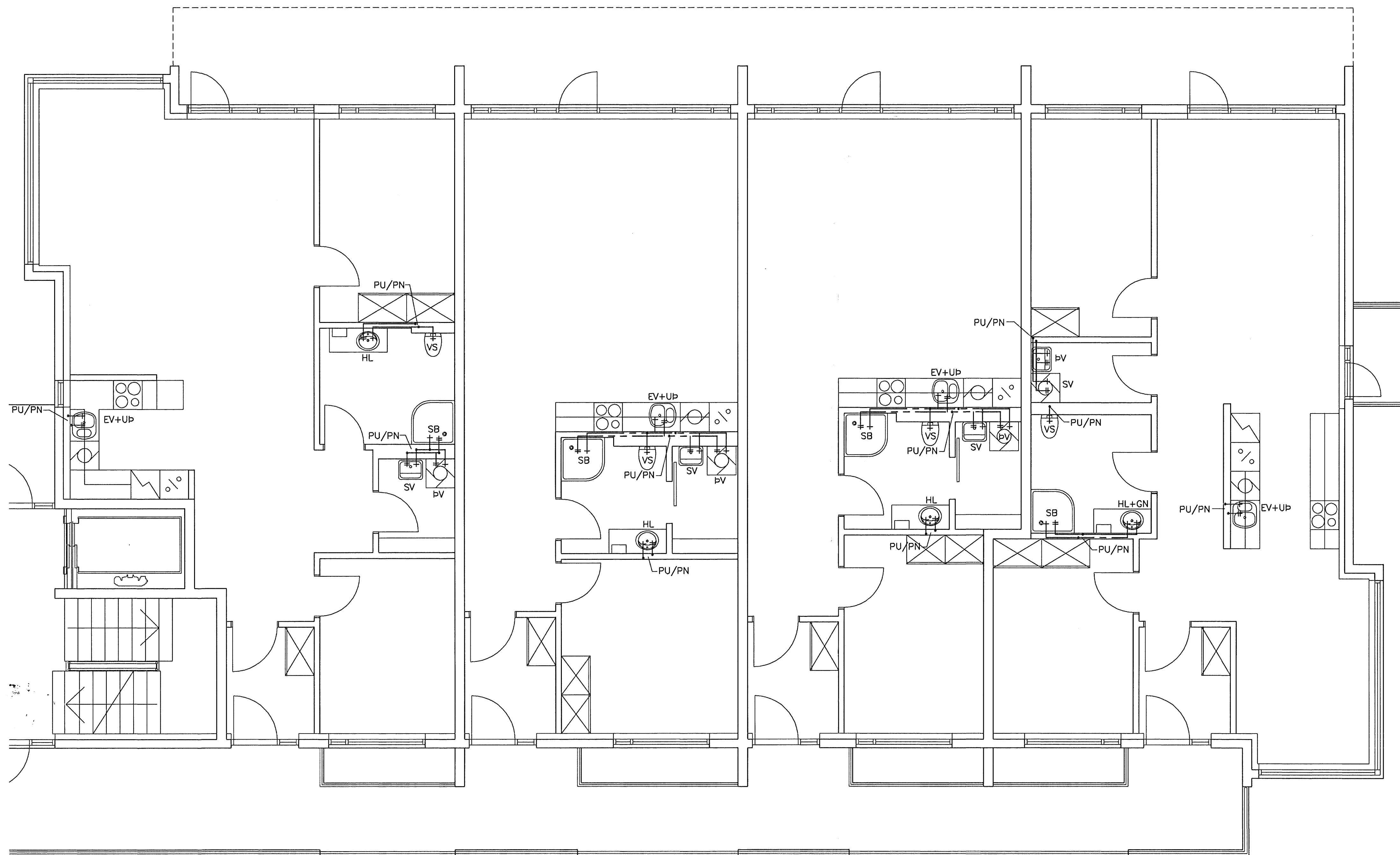
PN GRUNNMYND 2.-4. HÆÐ. 1:50
