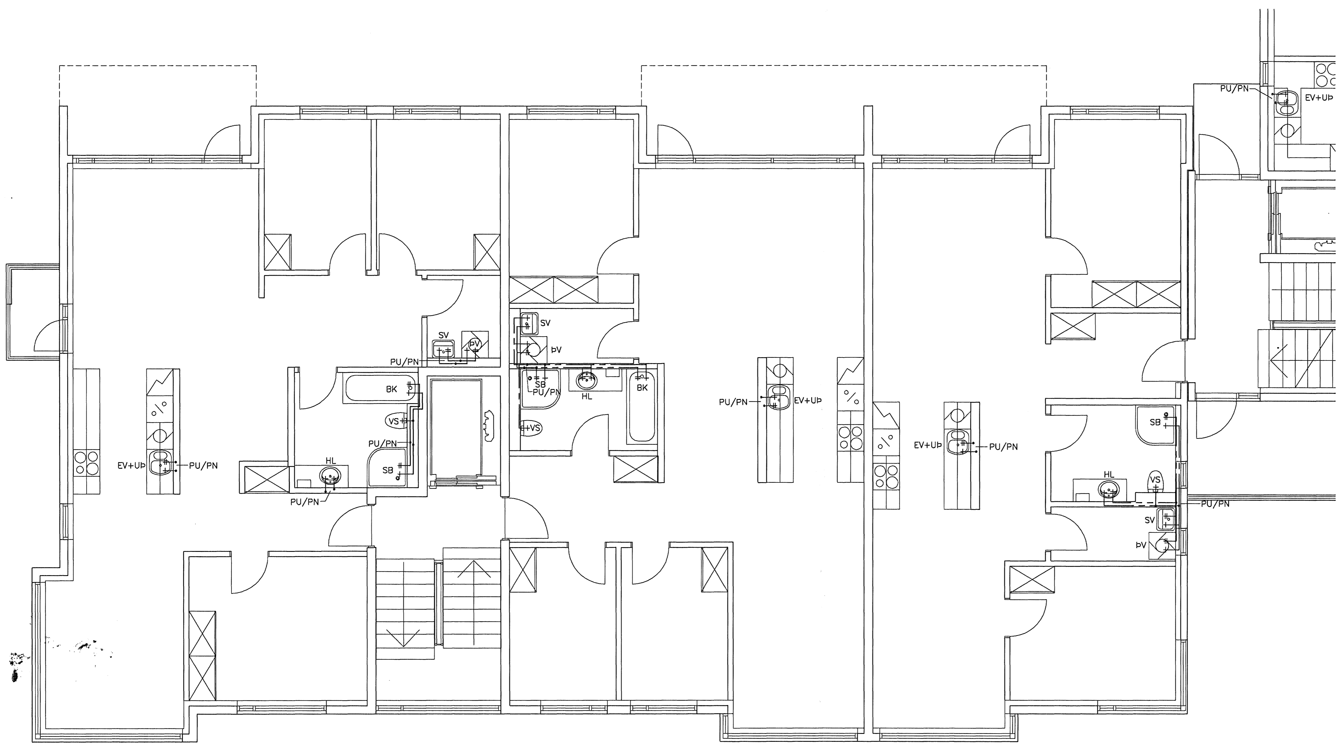
GRUNNMYND 2.-4. HÆÐ. 1:50
