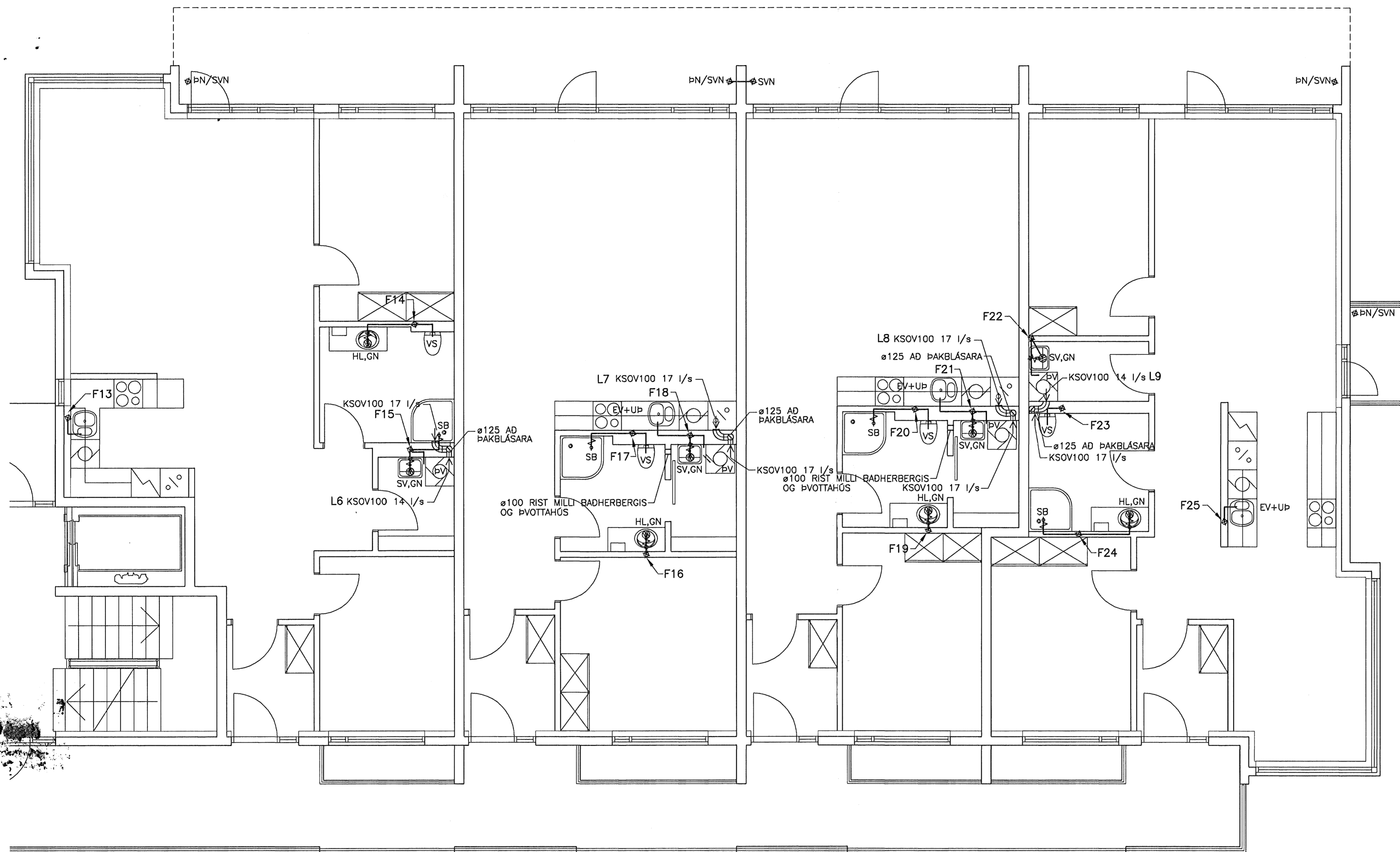
GRUNNMYND 2.HÆD. 1:50
