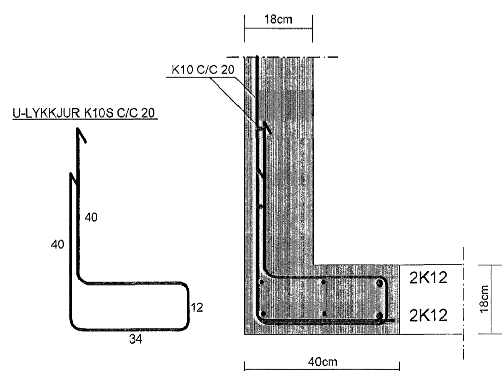
SNID 9-9 MKV. 1:10
