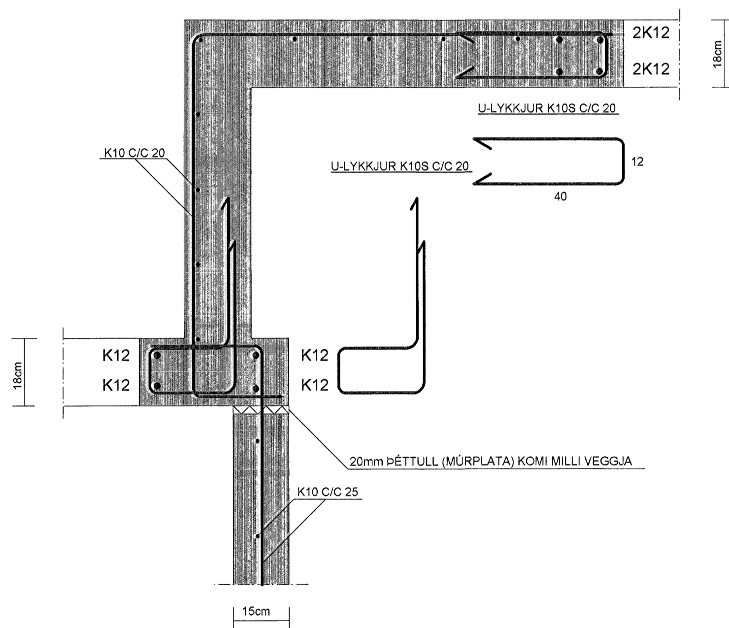
SNID 9-9 MKV. 1:10
