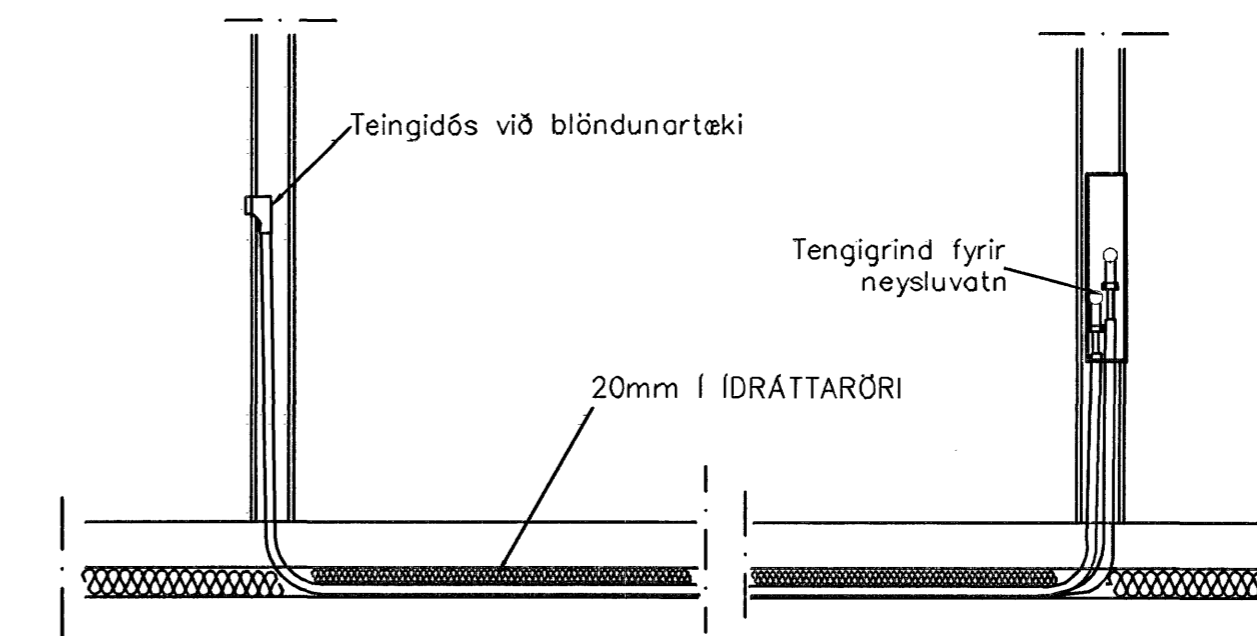
TENGING NEYSLUVATNSLAGNA 1:20
