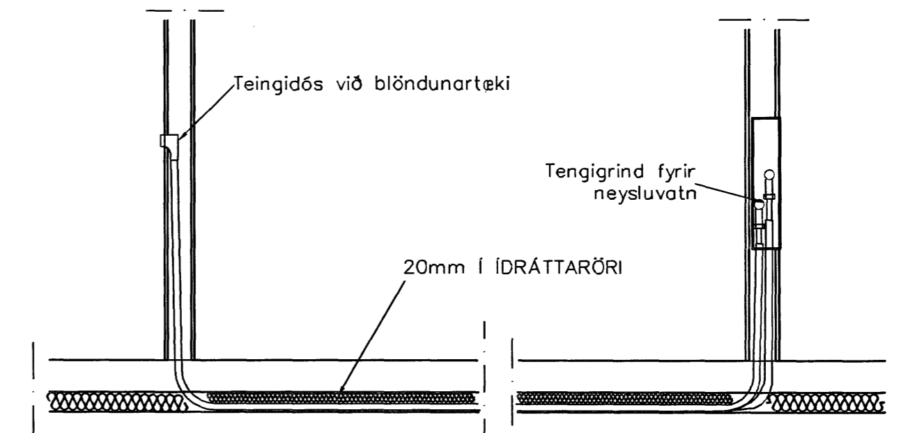
TENING NEYSLUVATNSLAGNA 1:20
