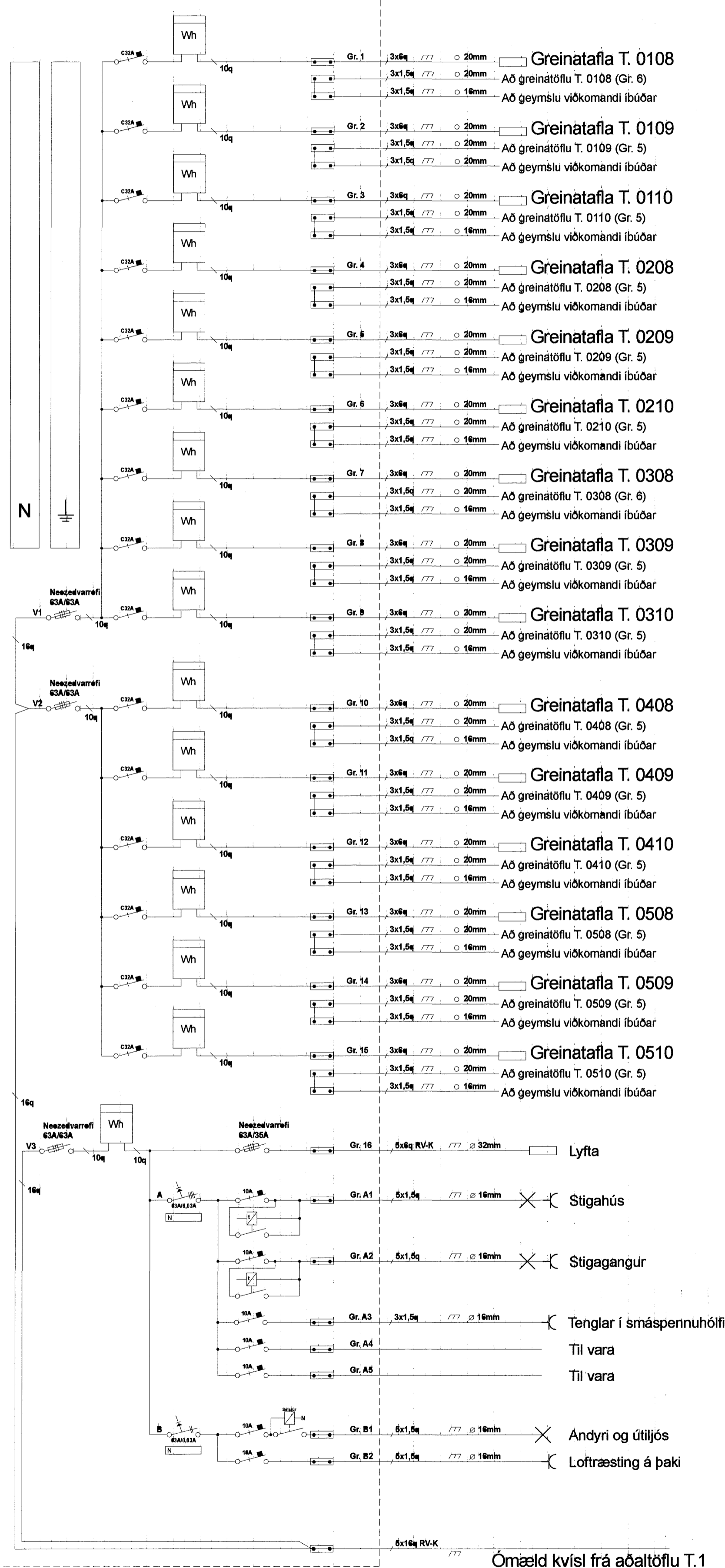
Einlínunmynd Töflu T.1.4 3/N ~ 400/230V
