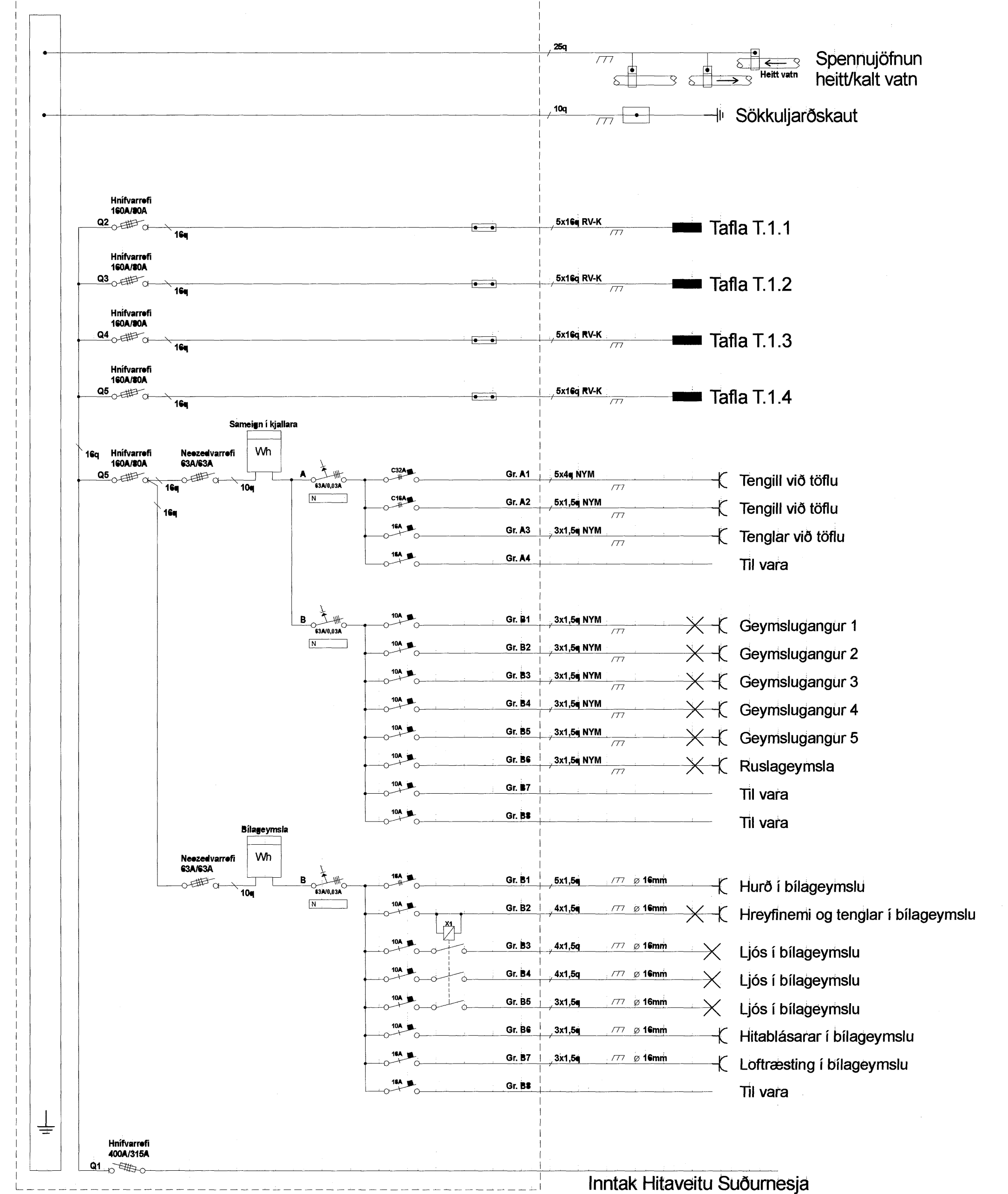
Einlínunmynd Töflu T.1 3/N ~ 400/230V
