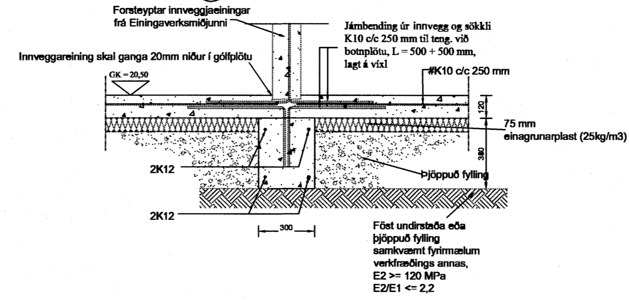
B3 Snið í sökkul 1:20
