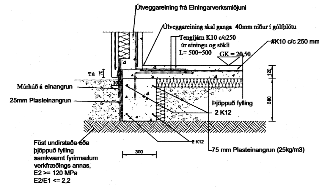
B2 Snið í sökkul 1:20
