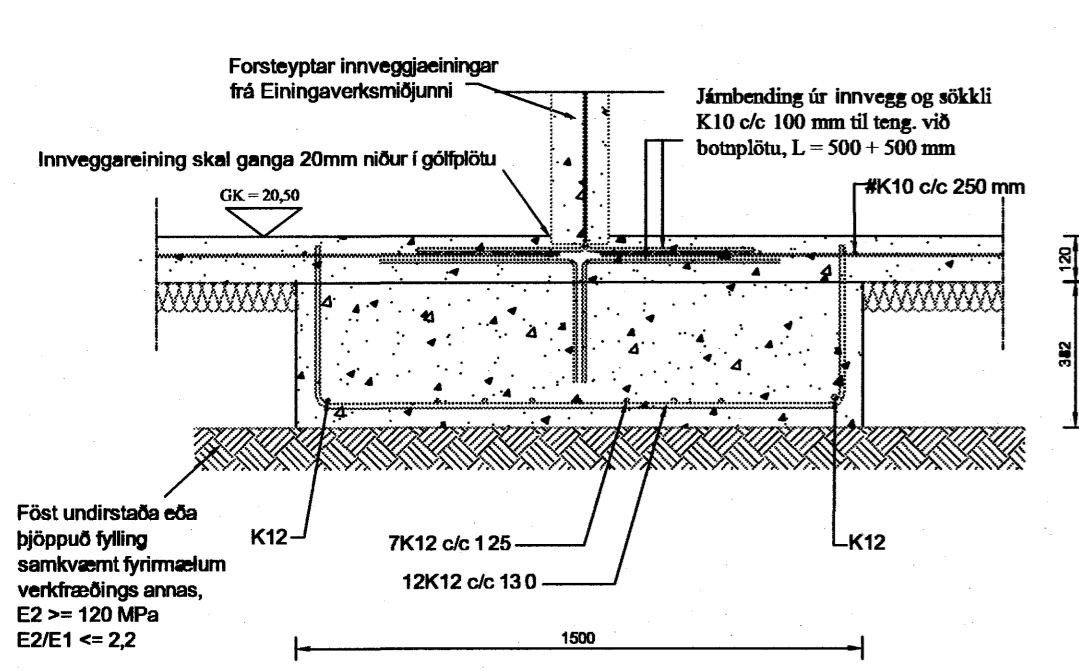
B4 Snið í sökkul 1:20
