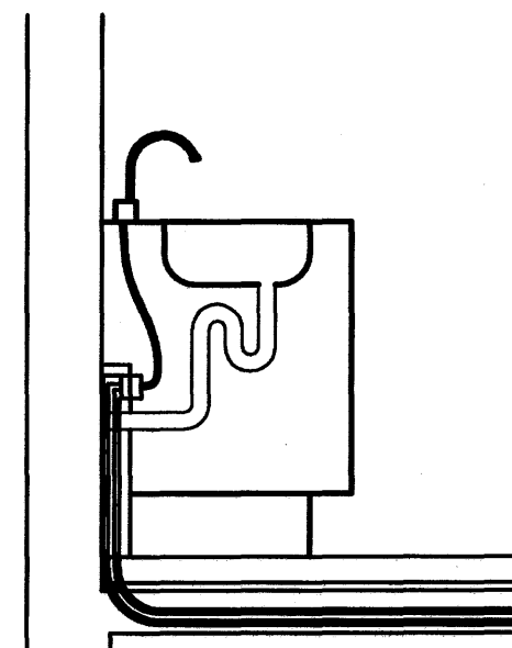
DÆMIGERÐUR FRÁGANGUR VIÐ HANDLAUGAR MKV. 2
