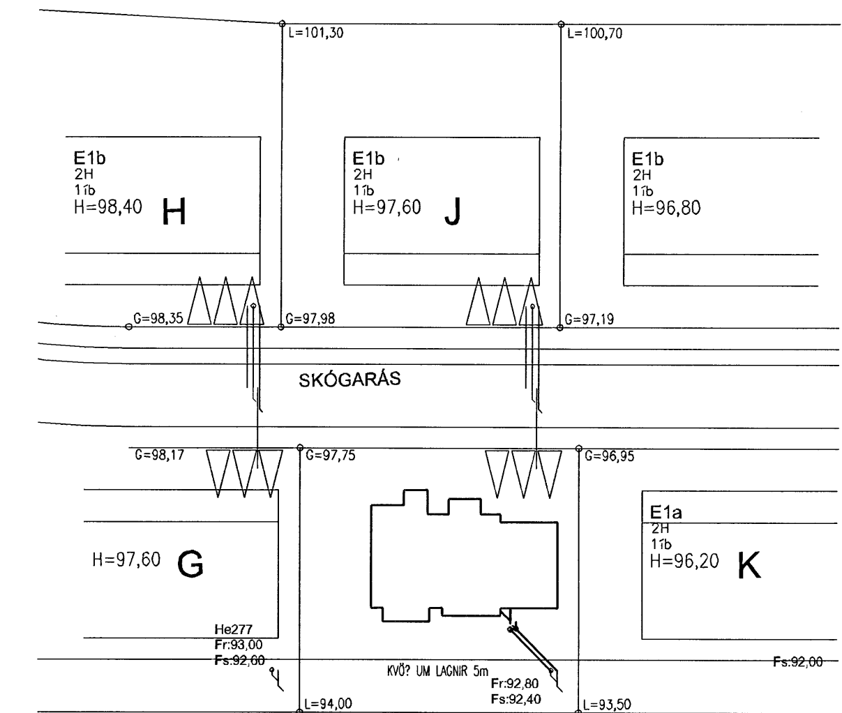
Afstöðumynd 1:500
