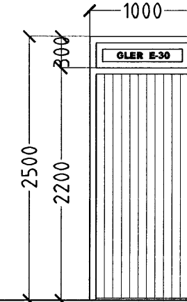
1 STK. SORP. HURÐ OPNAST HÆGRI ÚT. EI-C30 HURÐ.
