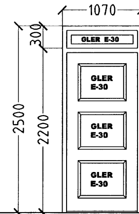
2 STK. VERSLUN/VINDFANG. HURÐ OPNAST VINSTRI INN. 1 STK. VERSLUN. HURÐ OPNAST HÆGRI INN.
