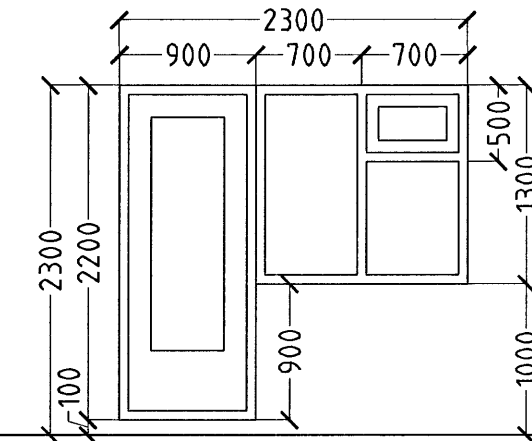
1 STK. HJÓN HURÐ OPNAST VINSTRI ÚT.
