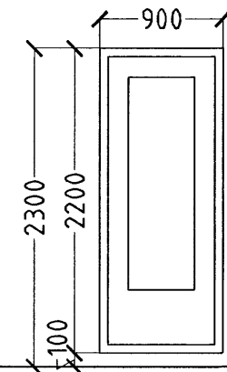
2 STK. STOFA. HURÐIR OPNAST HÆGRI ÚT.
