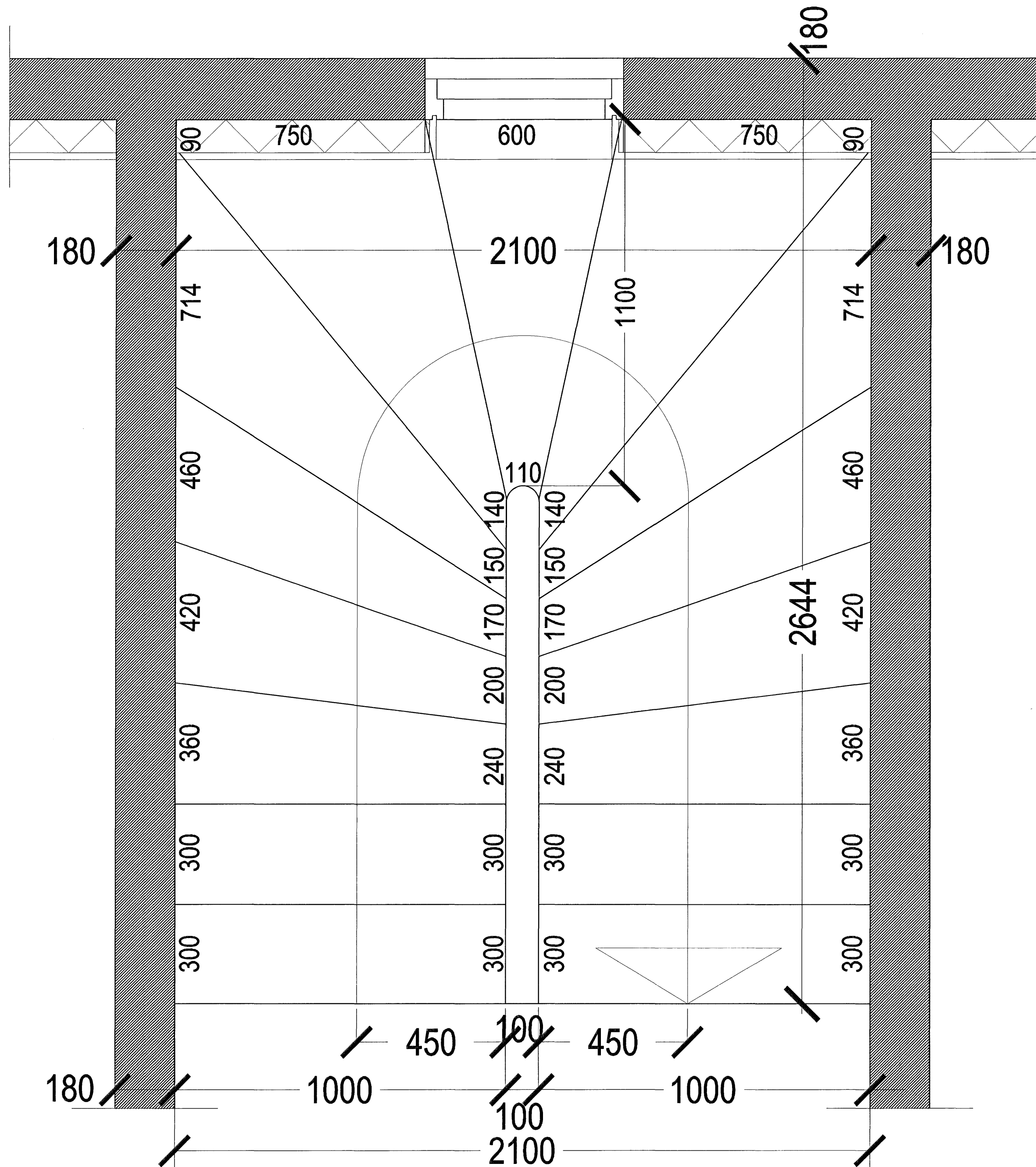
GRUNNMYND STIGI 2. og 3. HÆÐ, MKV. 1:10.
