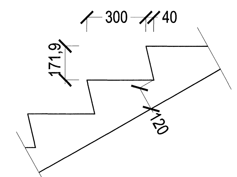
SNIÐ Í ÞREP, MKV. 1:10.
