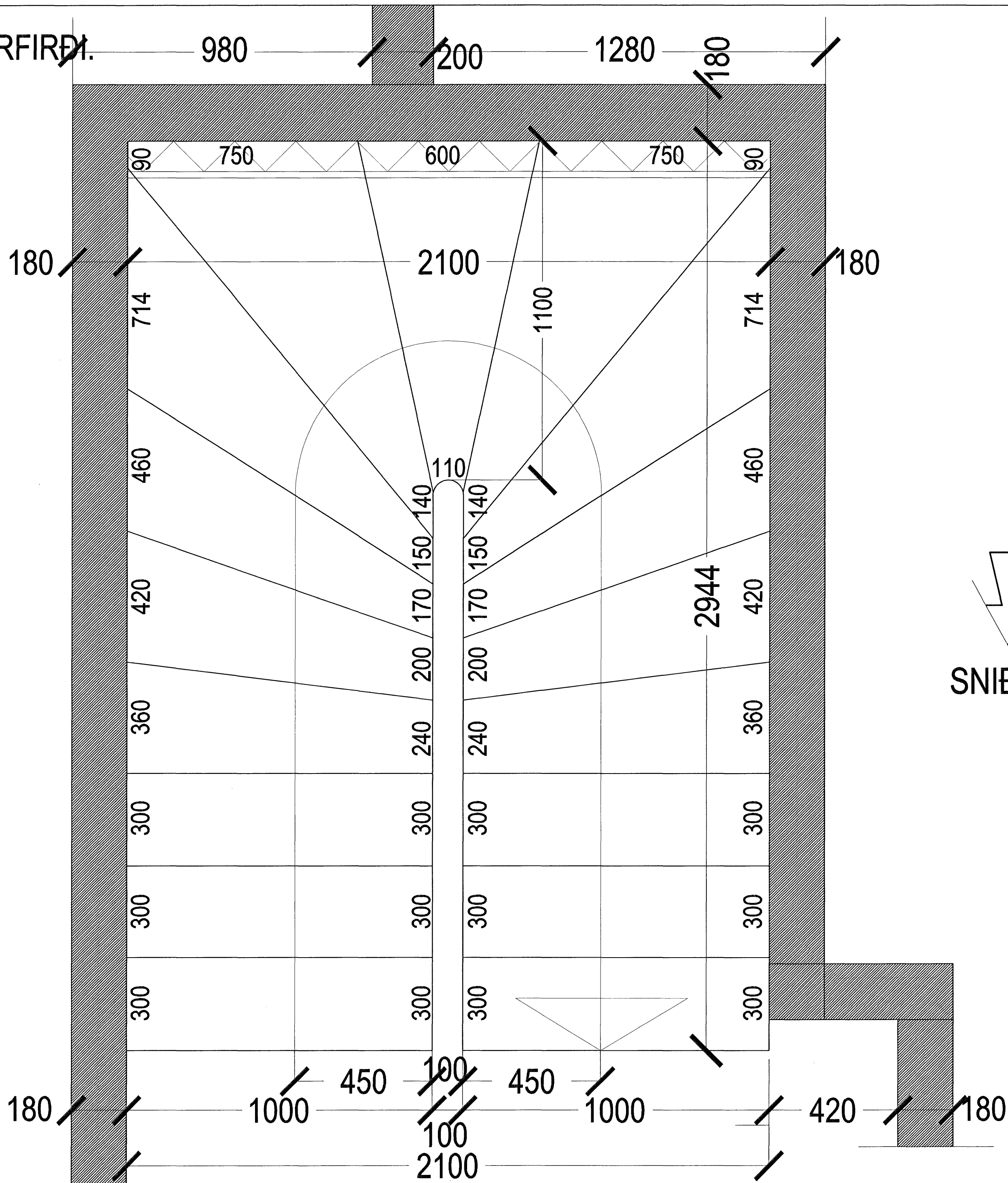
GRUNNMYND STIGI 1. HÆÐ, MKV. 1:10.
