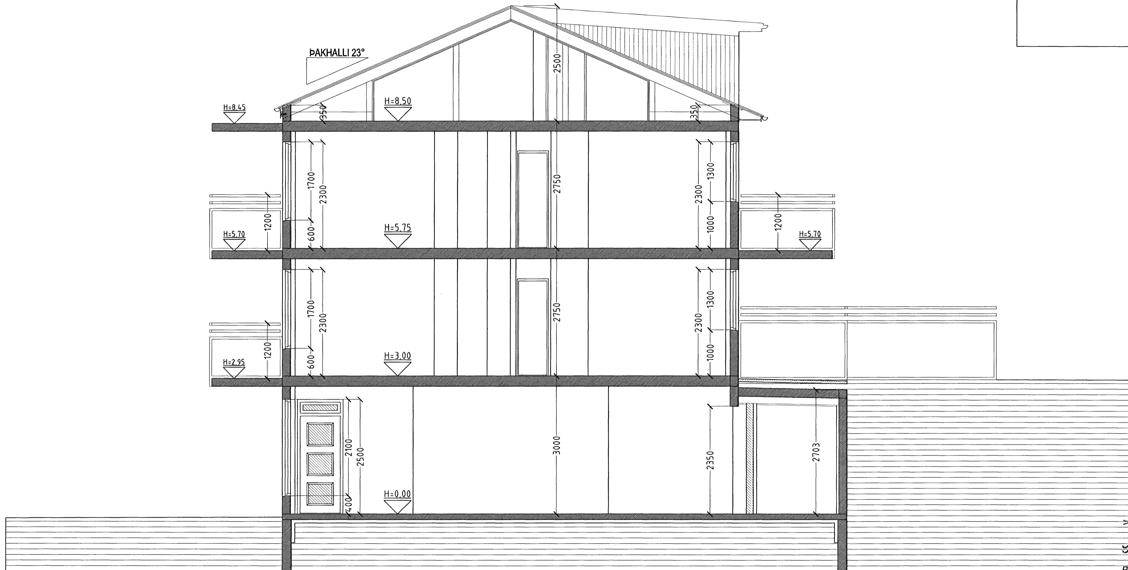
SNID C-C MKV. 1:50.
