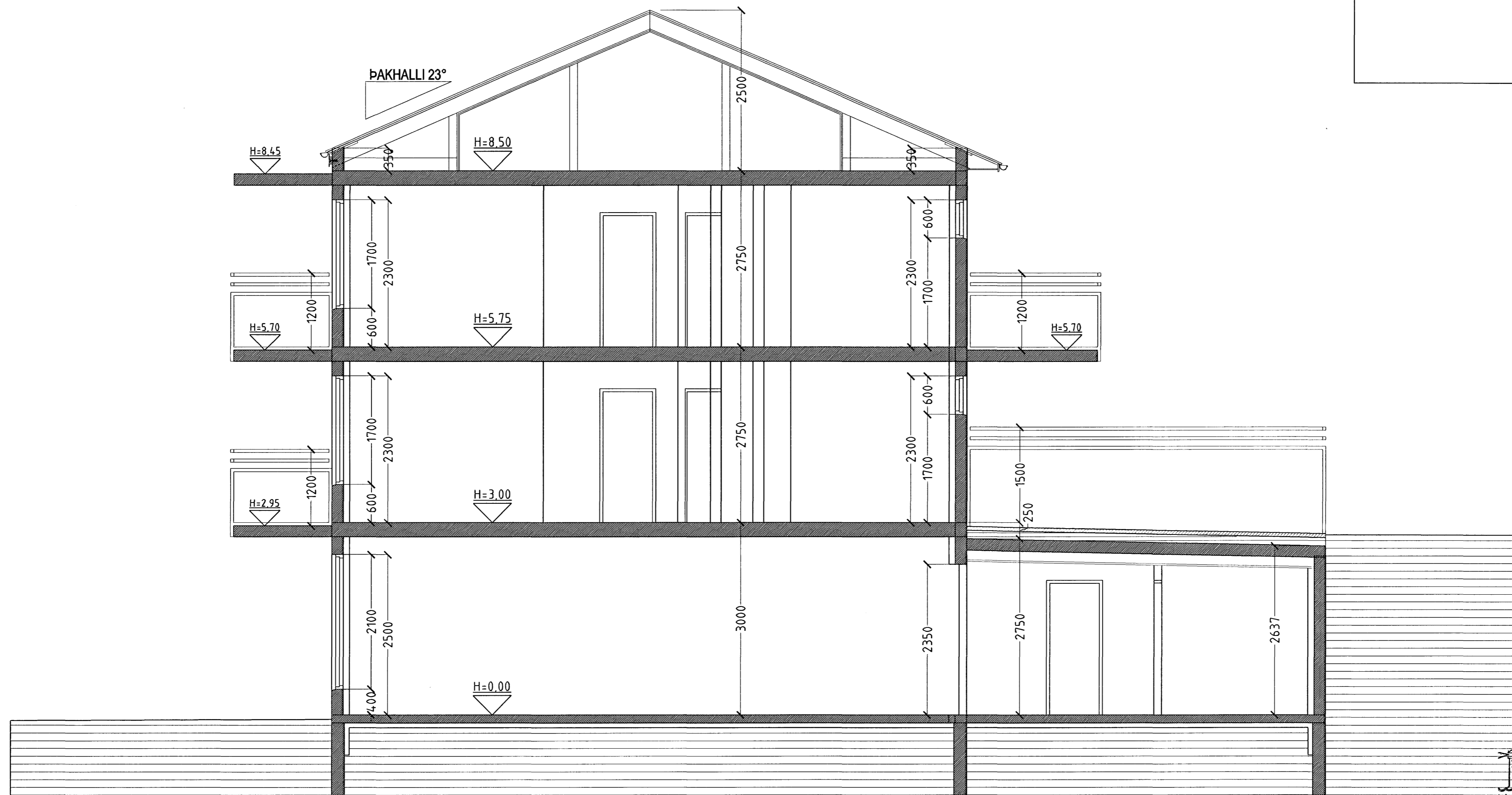
SNID A-A MKV. 1:50.
