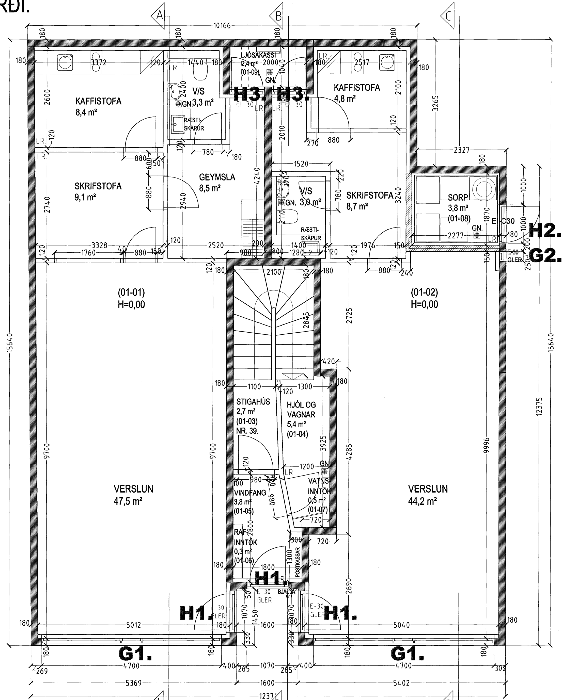
GRUNNMYND 1. HÆÐ MKV. 1:50.
