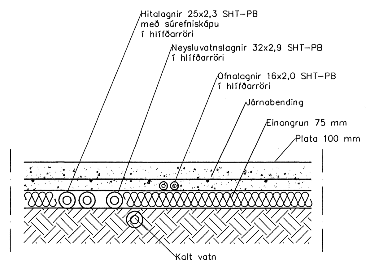
Hita- og Neysluvatnslagnir, Snið í botnplötu, 1:10
