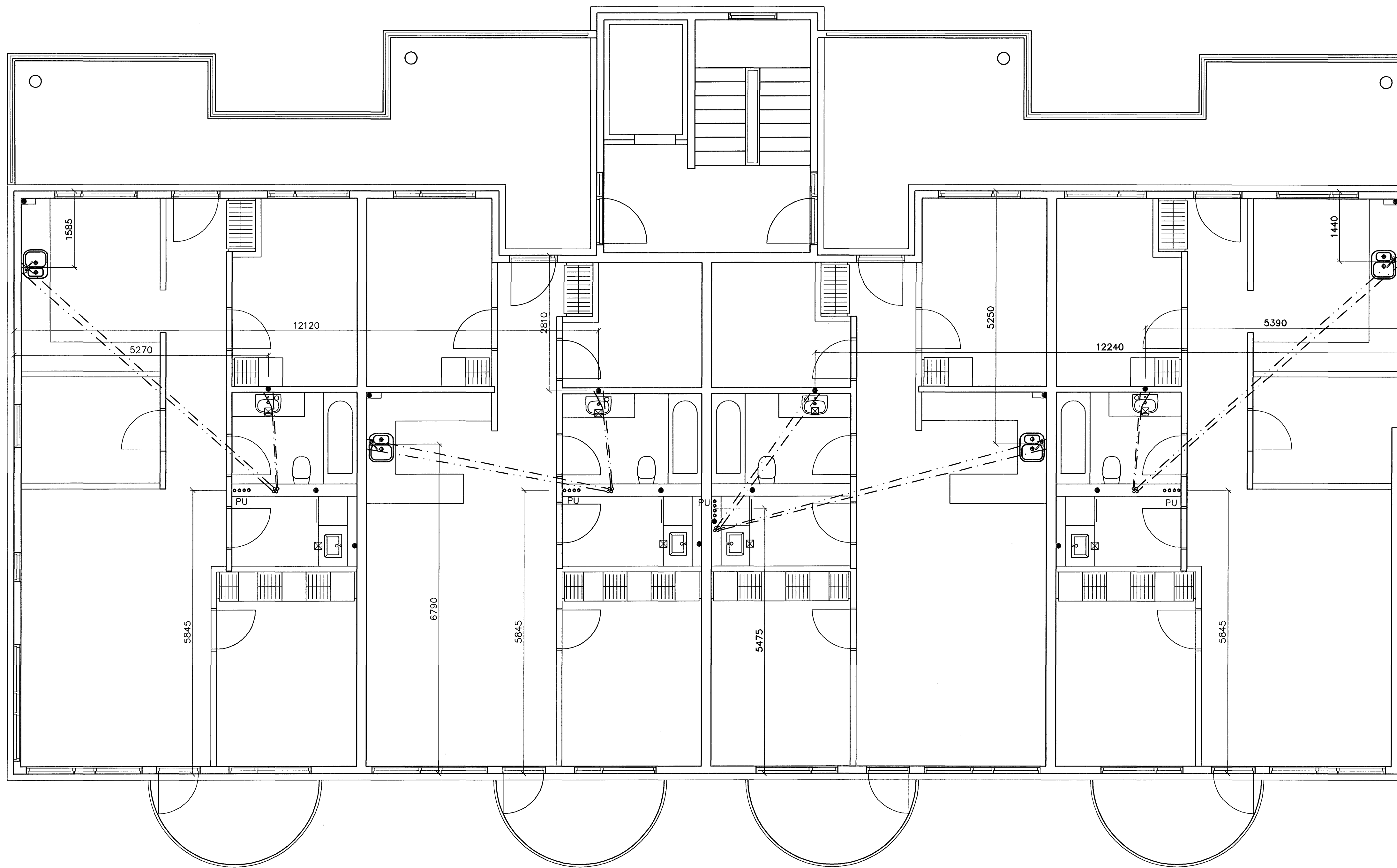
GRUNNMYND 2 HÆÐAR 1:50
