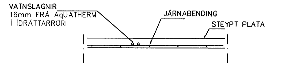
LAGNIR, SNIÐ, 1:20
