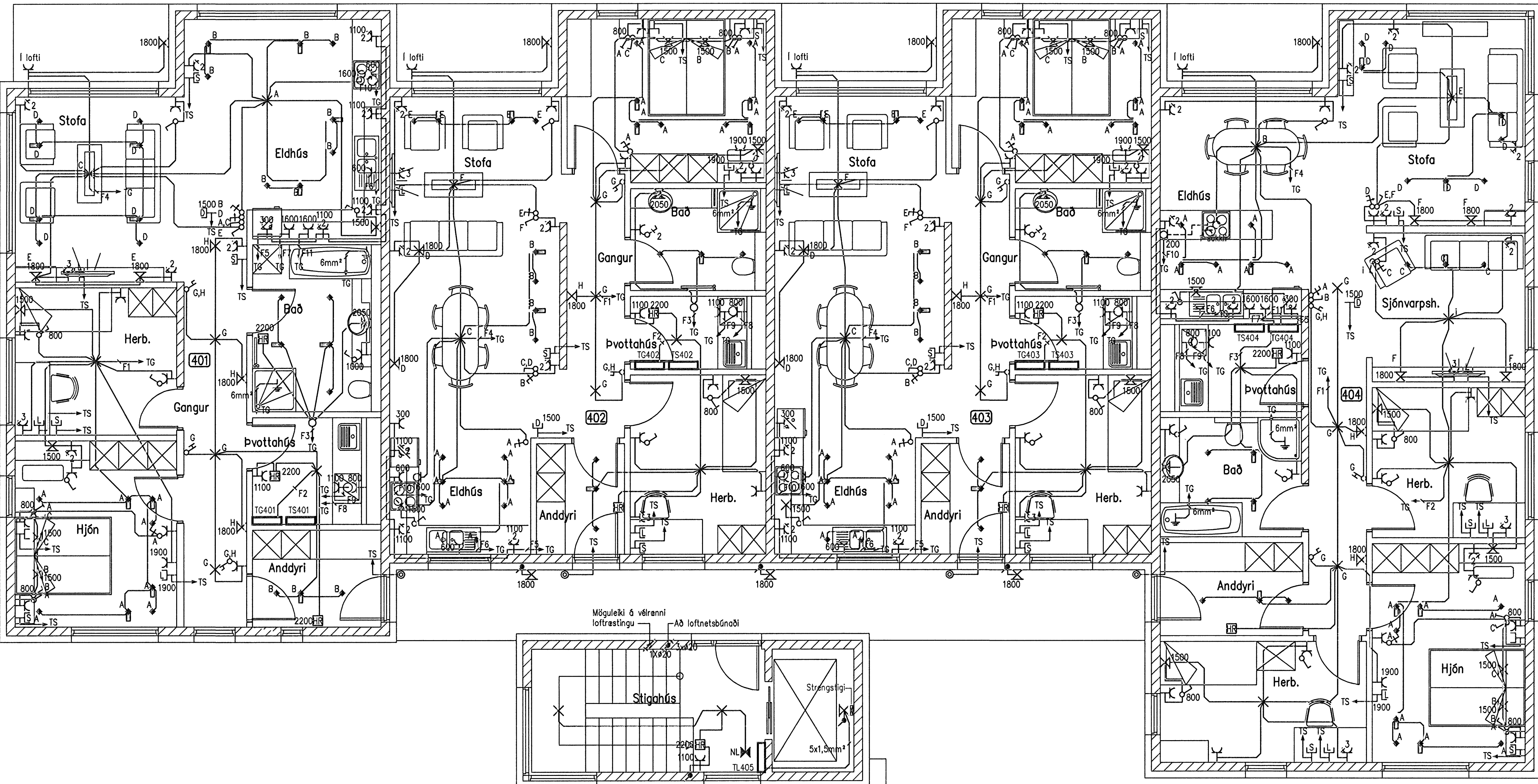
Grunnmynd 4.hæð 1:50
