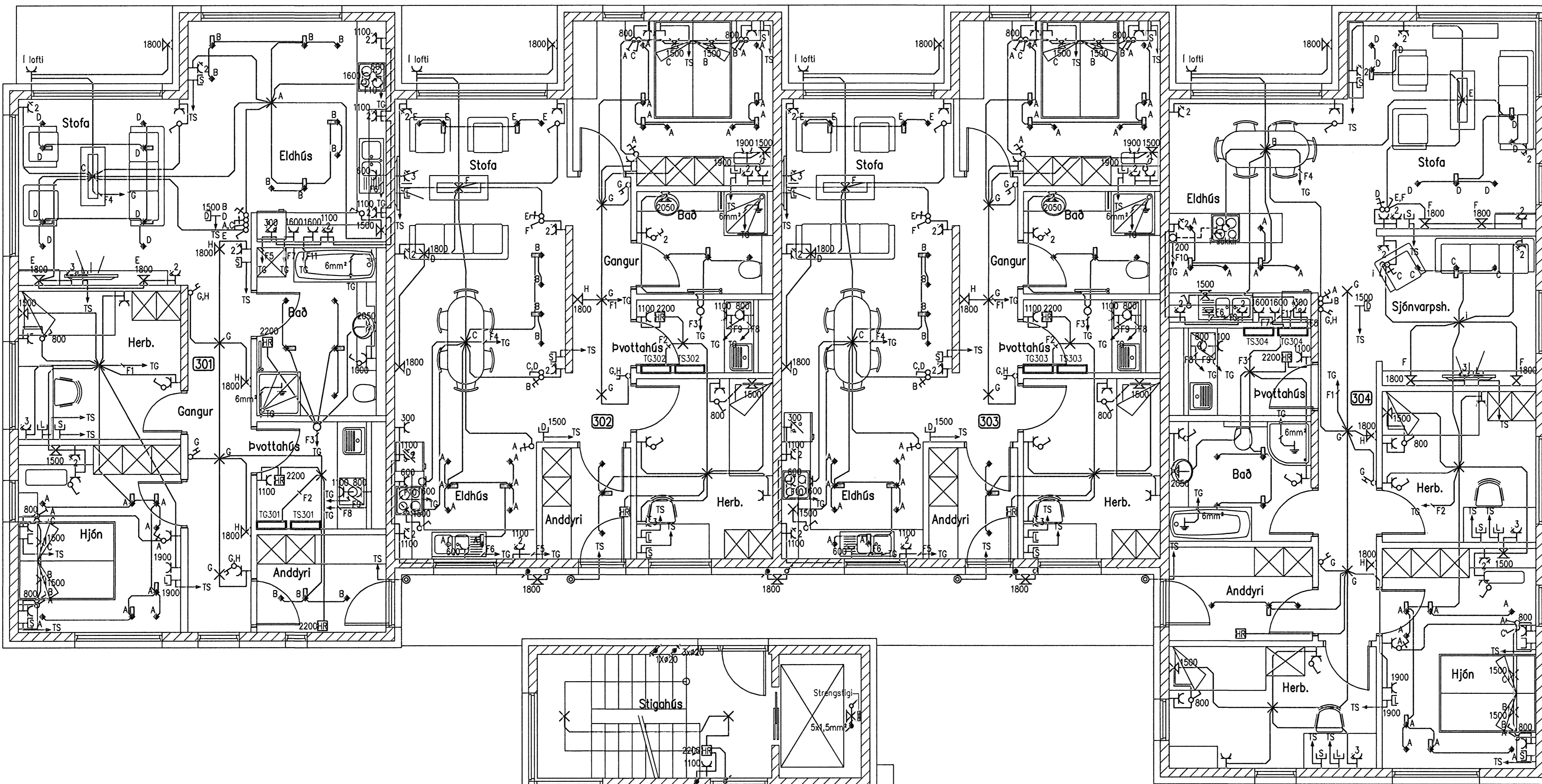
Grunnmynd 3.hæð 1:50
