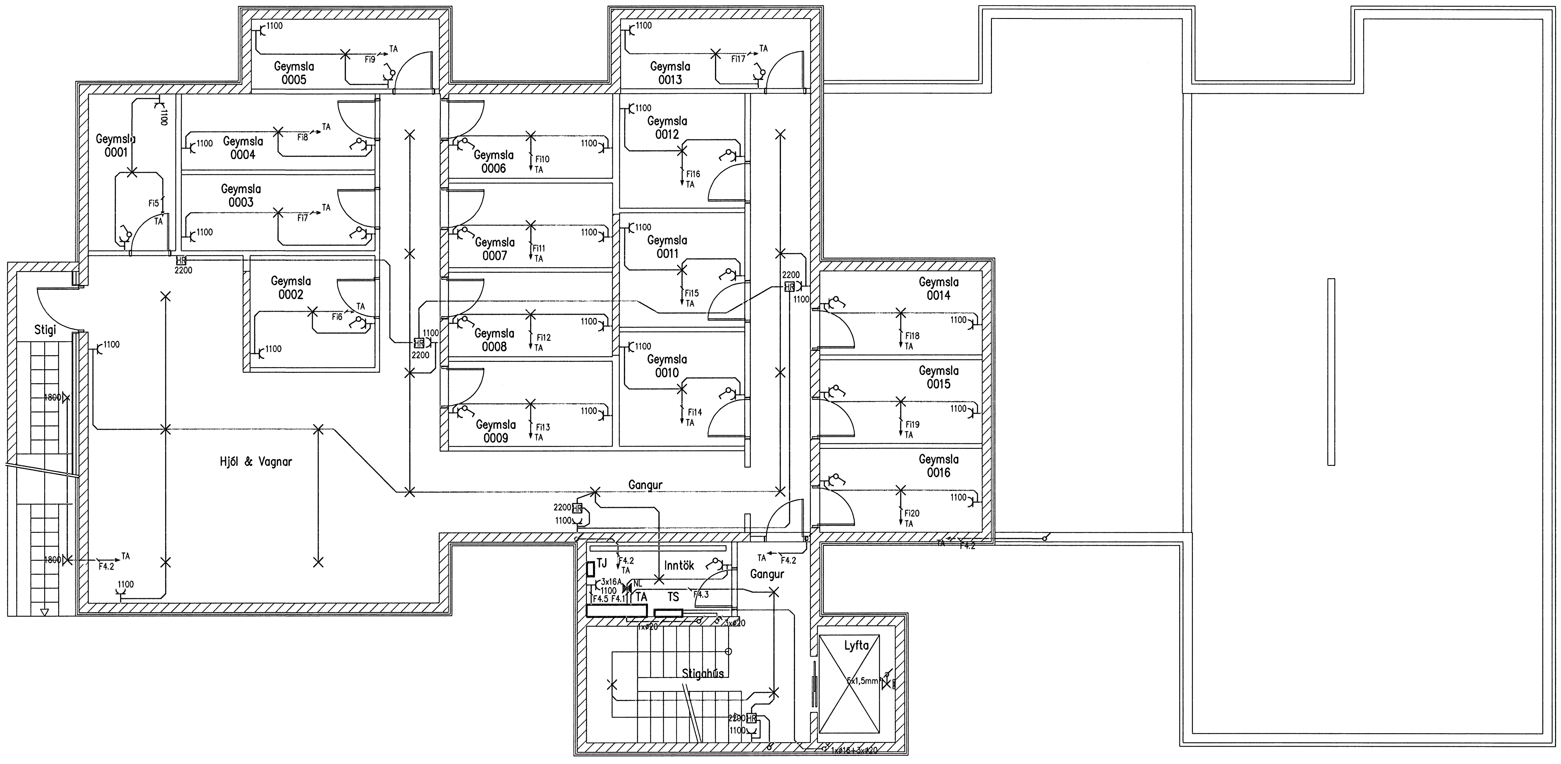
Grunnmynd kjallara 1:50
