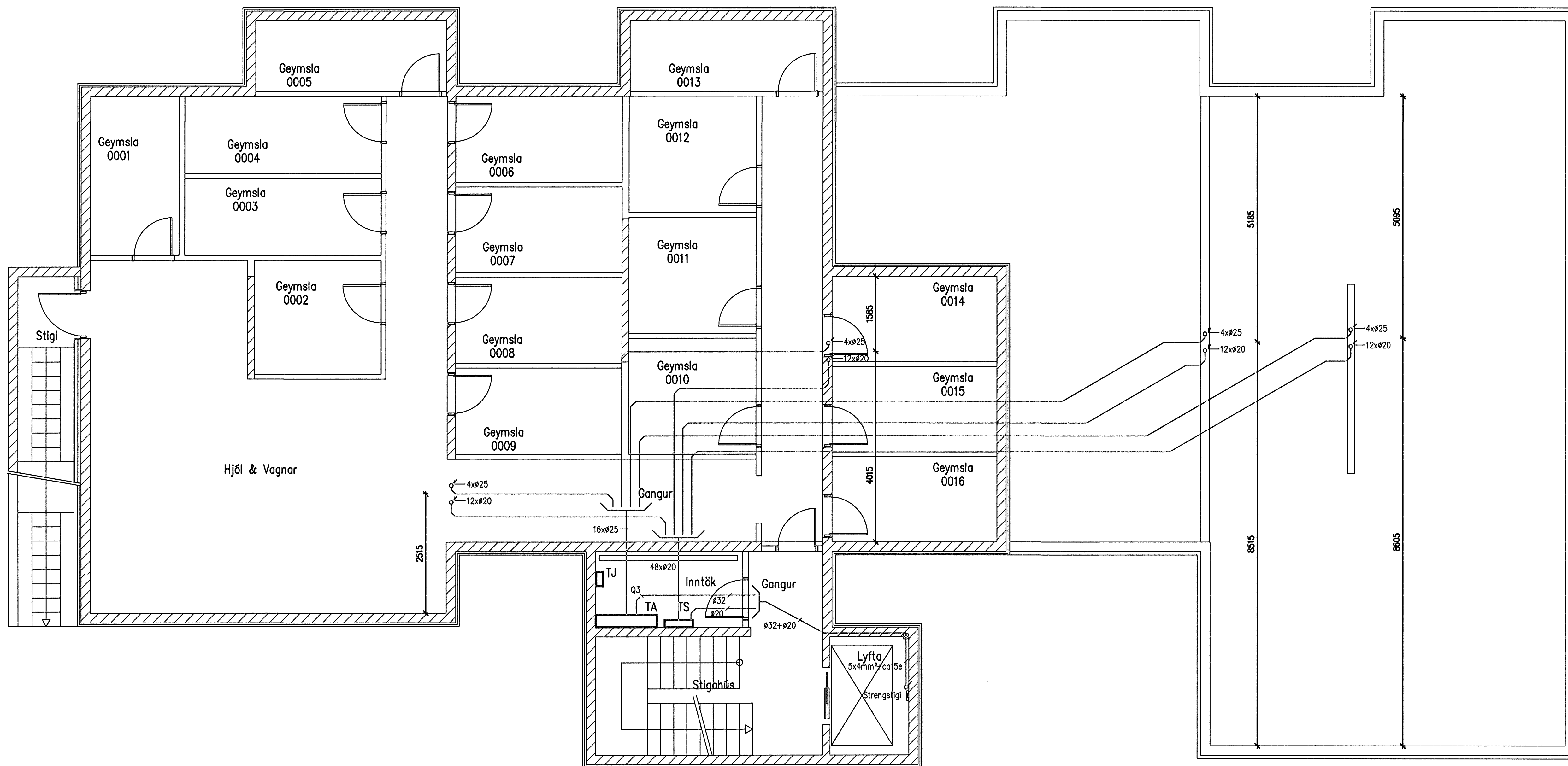
Grunnmynd kjallara 1:50
